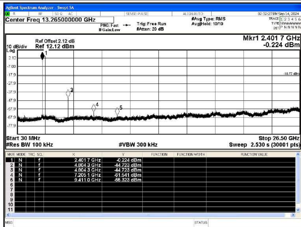
Tx. Spurious NVNT BLE 500Kbps 2402MHz Ant1 Emission
