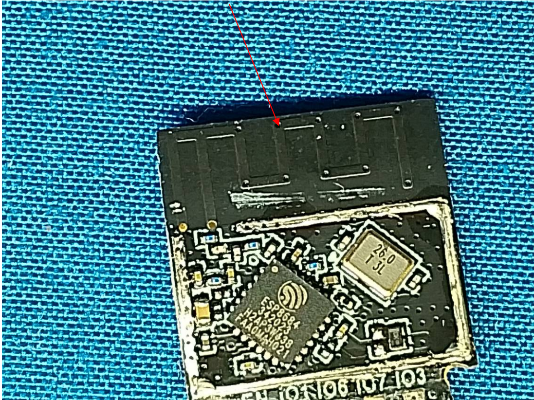
Bluetooth&Wifi Antenna
