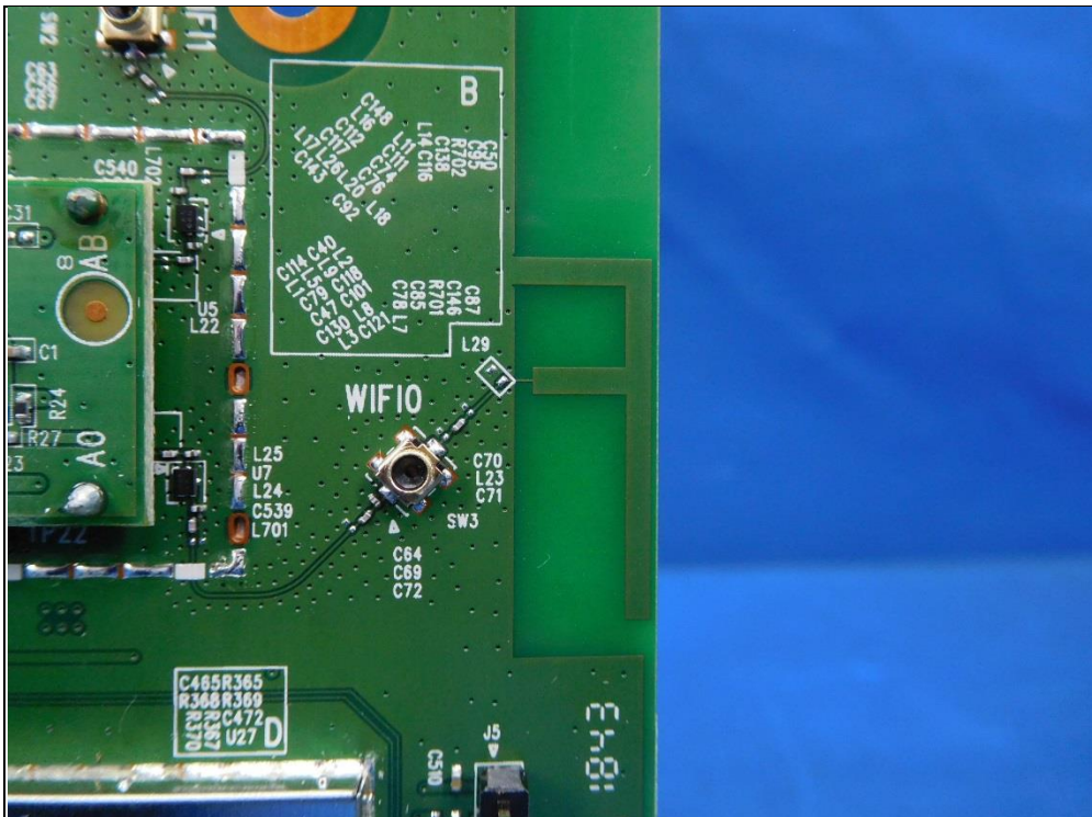
WLAN-ANT0
