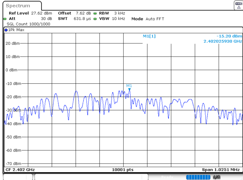
PSD NVNT BLE 2402MHz Ant1
