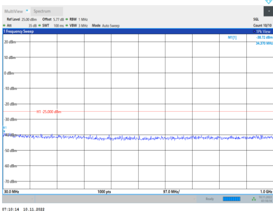
Band7-20MHz-QPSK-21350-1RB#0- Range1:30~1000MHz
