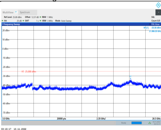
Band7-10MHz-QPSK-21100-1RB#0- Range3:3000~26500MHz
