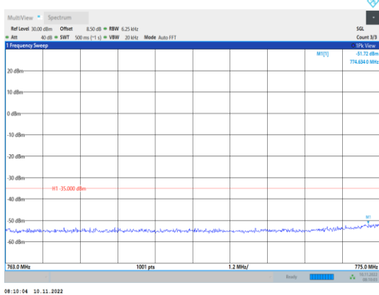
Band13-5MHz-QPSK-23230-1RB#0- Range3:763~775MHz
