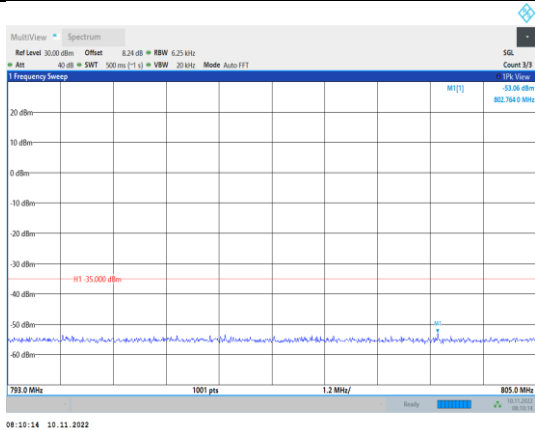
Band13-5MHz-QPSK-23230-1RB#0- Range4:793~805MHz
