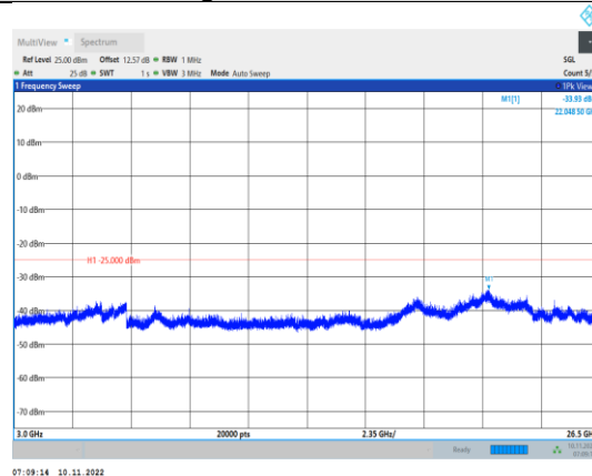
Band7-20MHz-QPSK-21100-1RB#0- Range3:3000~26500MHz
