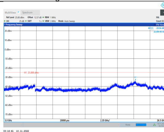
Band7-10MHz-QPSK-21400-1RB#0- Range3:3000~26500MHz
