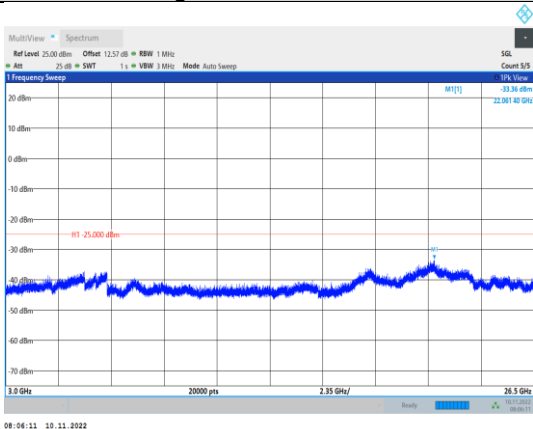
Band7-5MHz-QPSK-21425-1RB#0- Range3:3000~26500MHz
