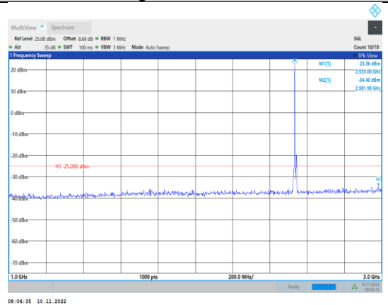
Band7-5MHz-QPSK-21100-1RB#0- Range2:1000~3000MHz
