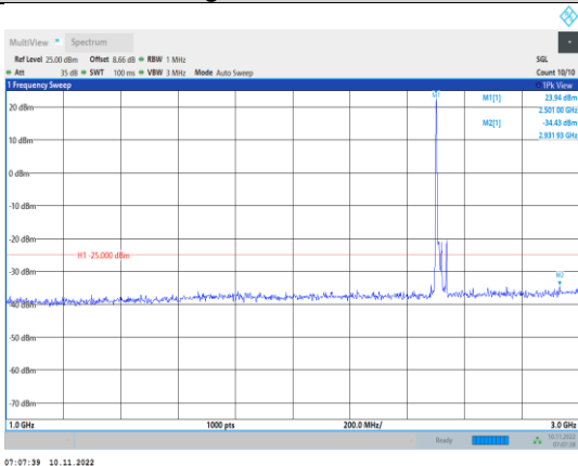
Band7-20MHz-QPSK-20850-1RB#0- Range2:1000~3000MHz
