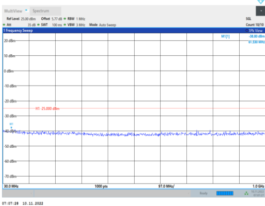
Band7-20MHz-QPSK-20850-1RB#0- Range1:30~1000MHz
