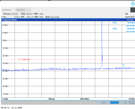
Band7-5MHz-QPSK-20775-1RB#0- Range2:1000~3000MHz
