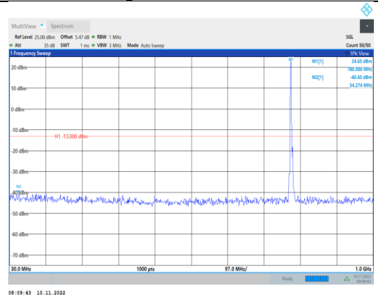
Band13-5MHz-QPSK-23230-1RB#0- Range1:30~1000MHz
