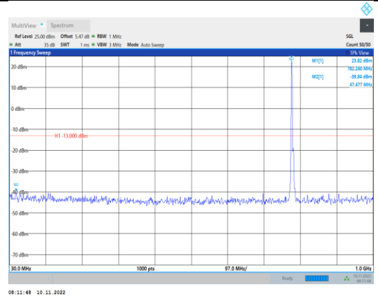
Band13-5MHz-QPSK-23255-1RB#0- Range1:30~1000MHz
