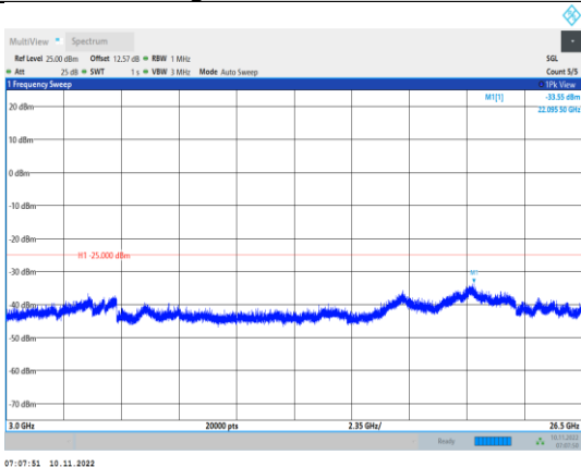
Band7-20MHz-QPSK-20850-1RB#0- Range3:3000~26500MHz
