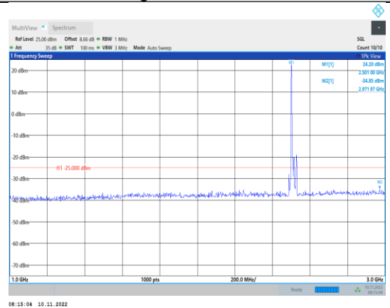
Band7-15MHz-QPSK-20825-1RB#0- Range2:1000~3000MHz
