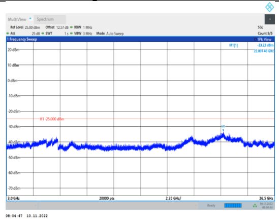
Band7-5MHz-QPSK-21100-1RB#0- Range3:3000~26500MHz
