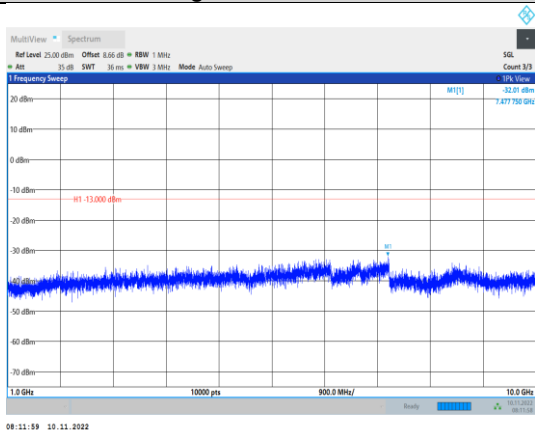
Band13-5MHz-QPSK-23255-1RB#0- Range2:1000~10000MHz
