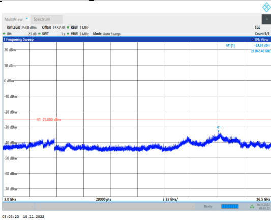
Band7-5MHz-QPSK-20775-1RB#0- Range3:3000~26500MHz
