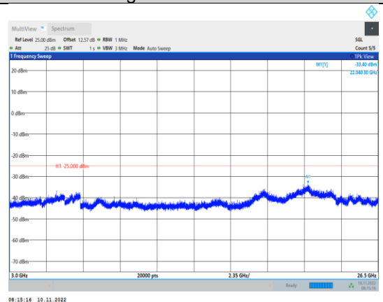
Band7-15MHz-QPSK-20825-1RB#0- Range3:3000~26500MHz
