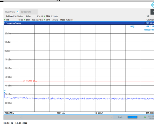
Band13-10MHz-QPSK-23230-1RB#0- Range4:793~805MHz
