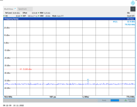
Band13-5MHz-QPSK-23255-1RB#0- Range3:763~775MHz
