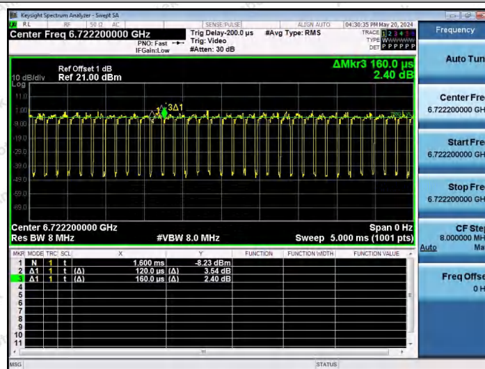
NTNV-11AX80SISO-Ant1-6705-484Tone-RU66
