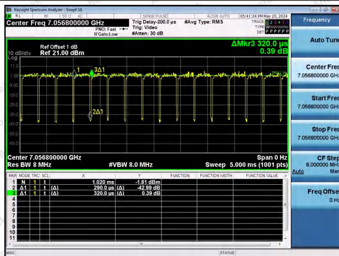
NTNV-11AX80SISO-Ant1-7025-106Tone-RU60
