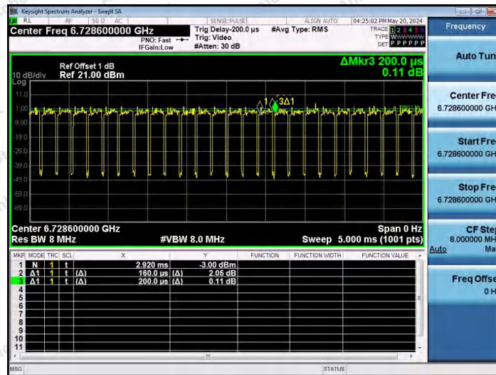
NTNV-11AX80SISO-Ant1-6705-242Tone-RU64
