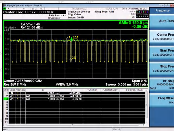
NTNV-11AX80SISO-Ant1-7025-484Tone-RU66
