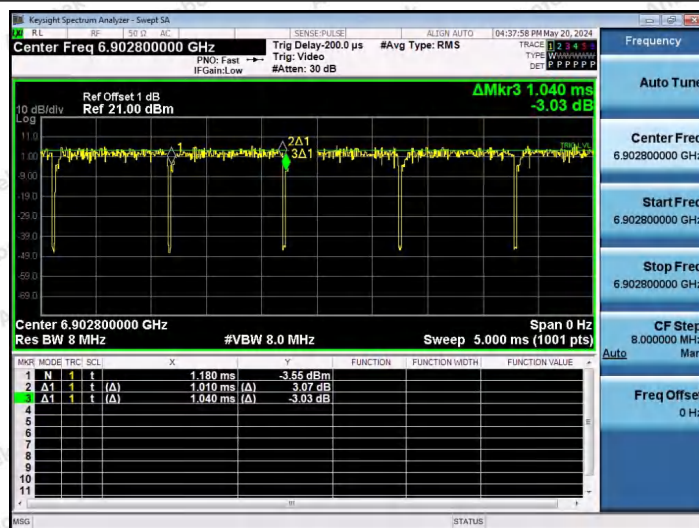
NTNV-11AX80SISO-Ant1-6865-26Tone-RU36
