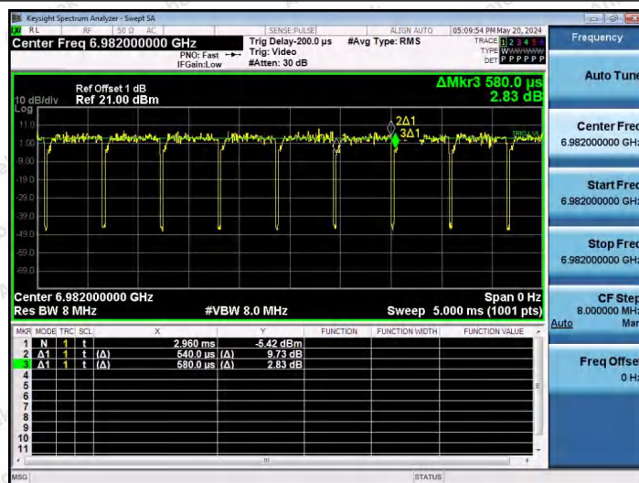
NTNV-11AX80SISO-Ant1-6945-52Tone-RU52
