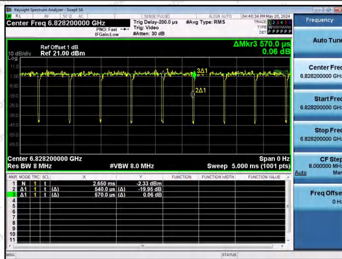
NTNV-11AX80SISO-Ant1-6865-52Tone-RU37
