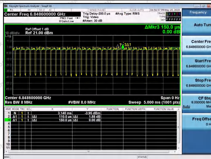
NTNV-11AX80SISO-Ant1-6865-484Tone-RU65
