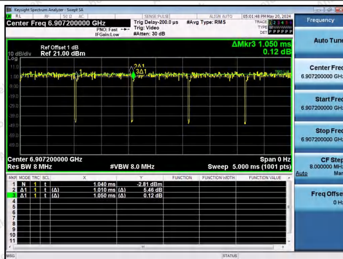
NTNV-11AX80SISO-Ant1-6945-26Tone-RU0
