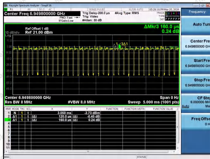
NTNV-11AX80SISO-Ant1-6945-484Tone-RU66
