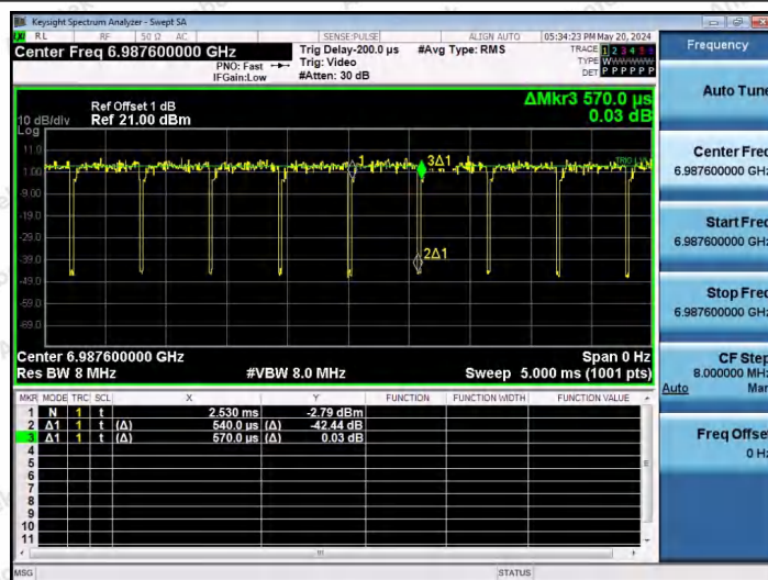
NTNV-11AX80SISO-Ant1-7025-52Tone-RU37
