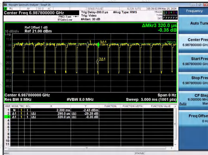
NTNV-11AX80SISO-Ant1-7025-106Tone-RU53
