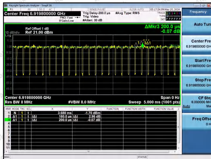
NTNV-11AX80SISO-Ant1-6945-242Tone-RU61
