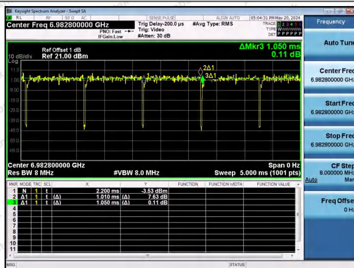
NTNV-11AX80SISO-Ant1-6945-26Tone-RU36
