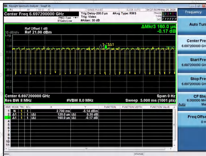
NTNV-11AX80SISO-Ant1-6705-484Tone-RU65
