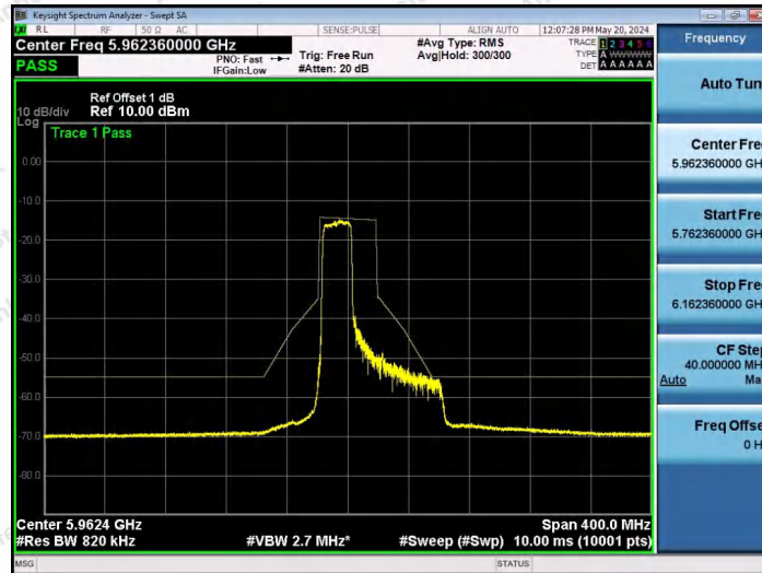
NTNV-11AX80SISO-Ant1-5985-242Tone-RU61-PASS
