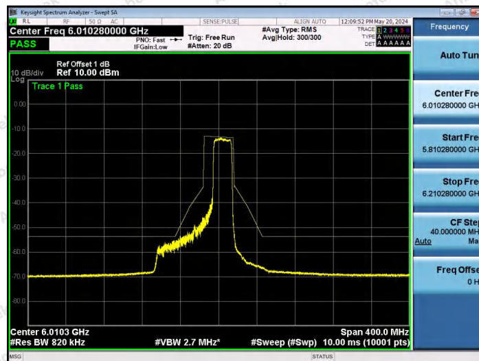
NTNV-11AX80SISO-Ant1-5985-242Tone-RU64-PASS
