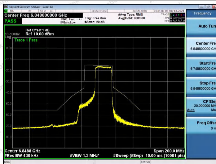
NTNV-11AX40SISO-Ant1-6845-242Tone-RU62-PASS
