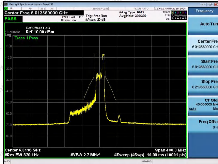
NTNV-11AX80SISO-Ant1-5985-52Tone-RU52-PASS
