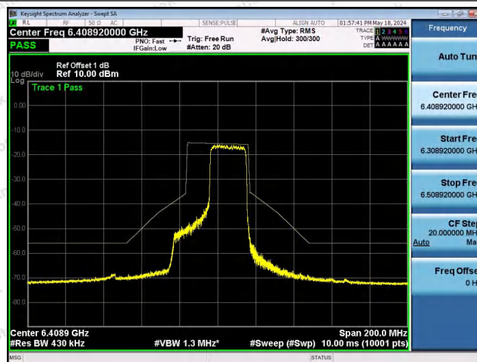
NTNV-11AX40SISO-Ant1-6405-242Tone-RU62-PASS
