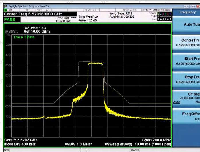
NTNV-11AX40SISO-Ant1-6525-242Tone-RU62-PASS
