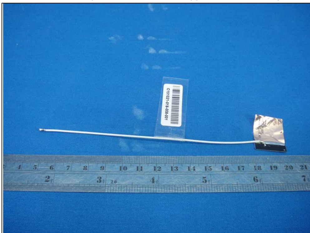
Antenna Set 7 (Brand: WNC / P/N: Chain (1): P/N: 1415-04LQ000)
