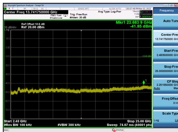
,Plot 4,2483.5MHz~25000MHz-802.11b
