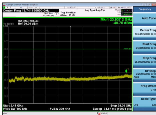
,Plot 4,2483.5MHz~25000MHz-802.11b
