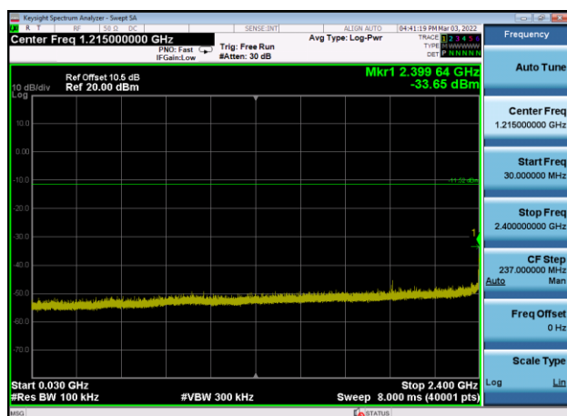
,Plot 3,30MHz~2400MHz-802.11b,2462MHz
