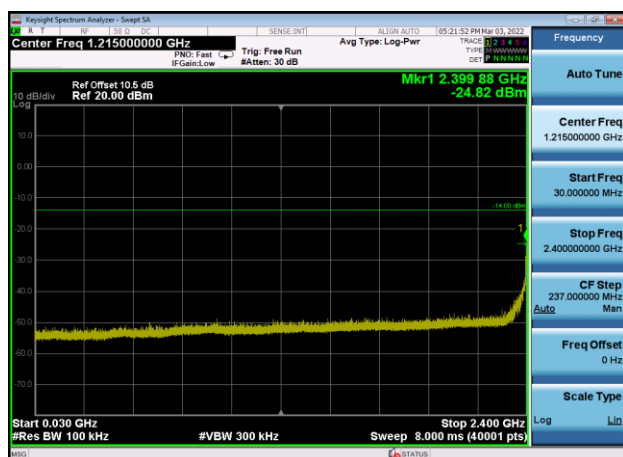
,Plot 3,30MHz~2400MHz-802.11g,2462MHz
