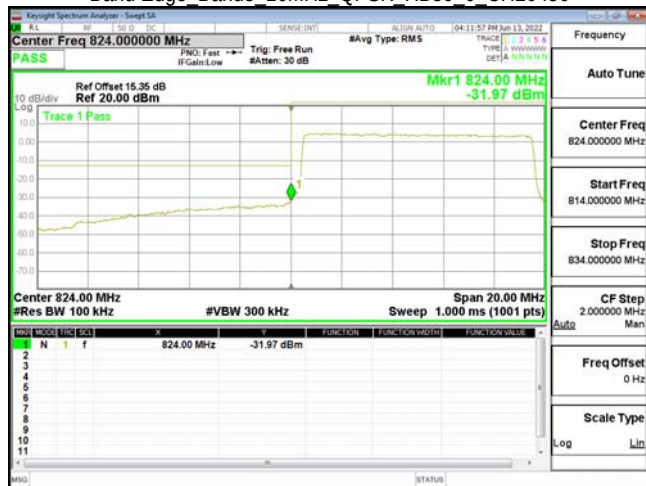
Band Edge Band5 10MHz QPSK RB50 0 CH20450
