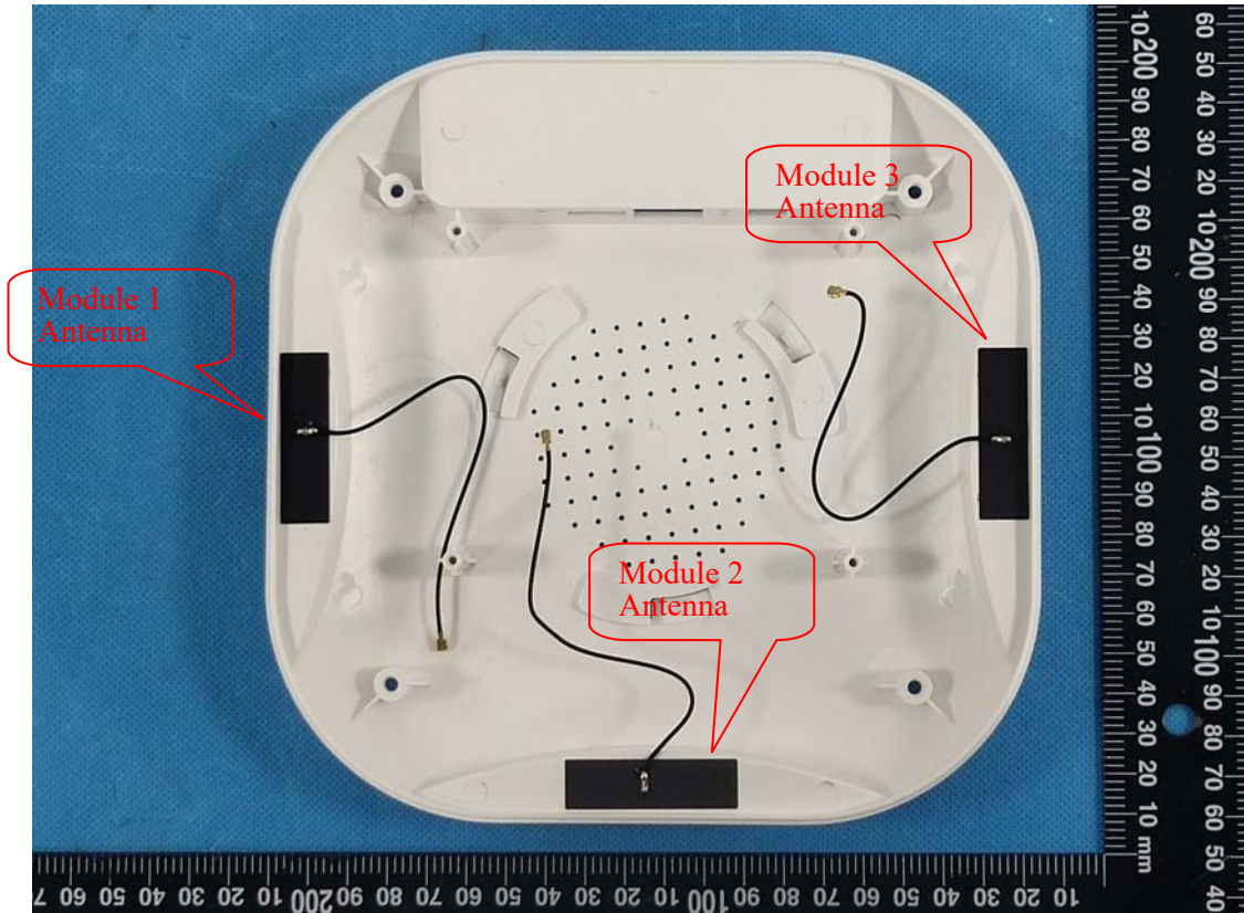
Module 3 Antenna
