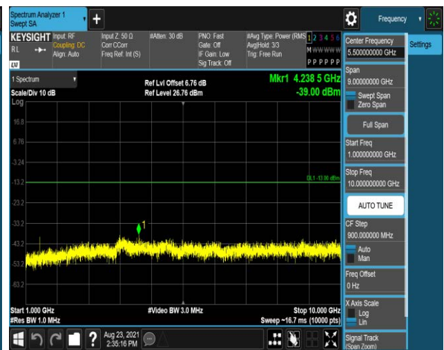
Band12-1.4MHz-QPSK-23095:1000~10000MHz
