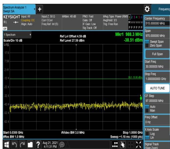
Band2-1.4MHz-QPSK-19193:30~1000MHz
