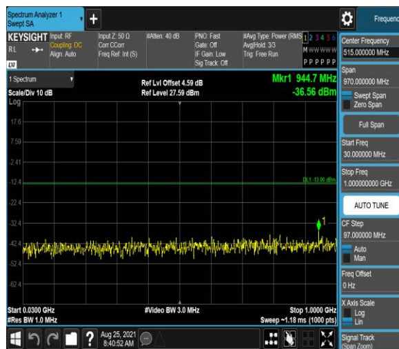
Band4-1.4MHz-QPSK-20393:30~1000MHz
