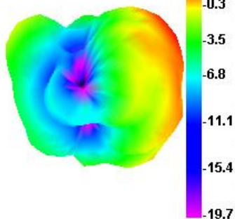
400.000MHz E1
