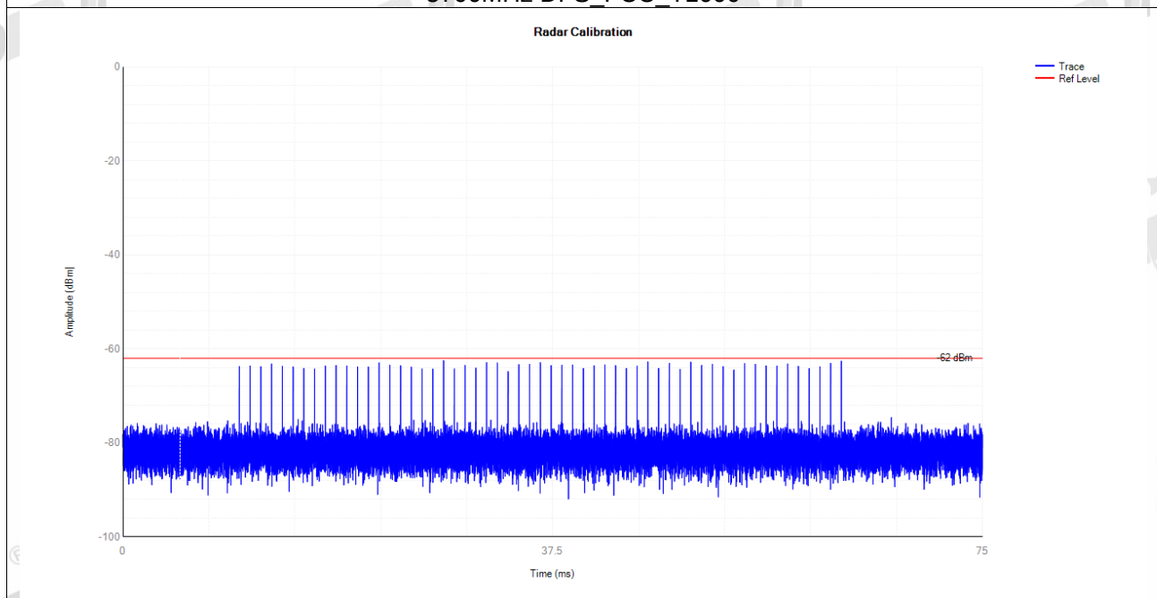
5700MHz DFS_FCC_T2000
