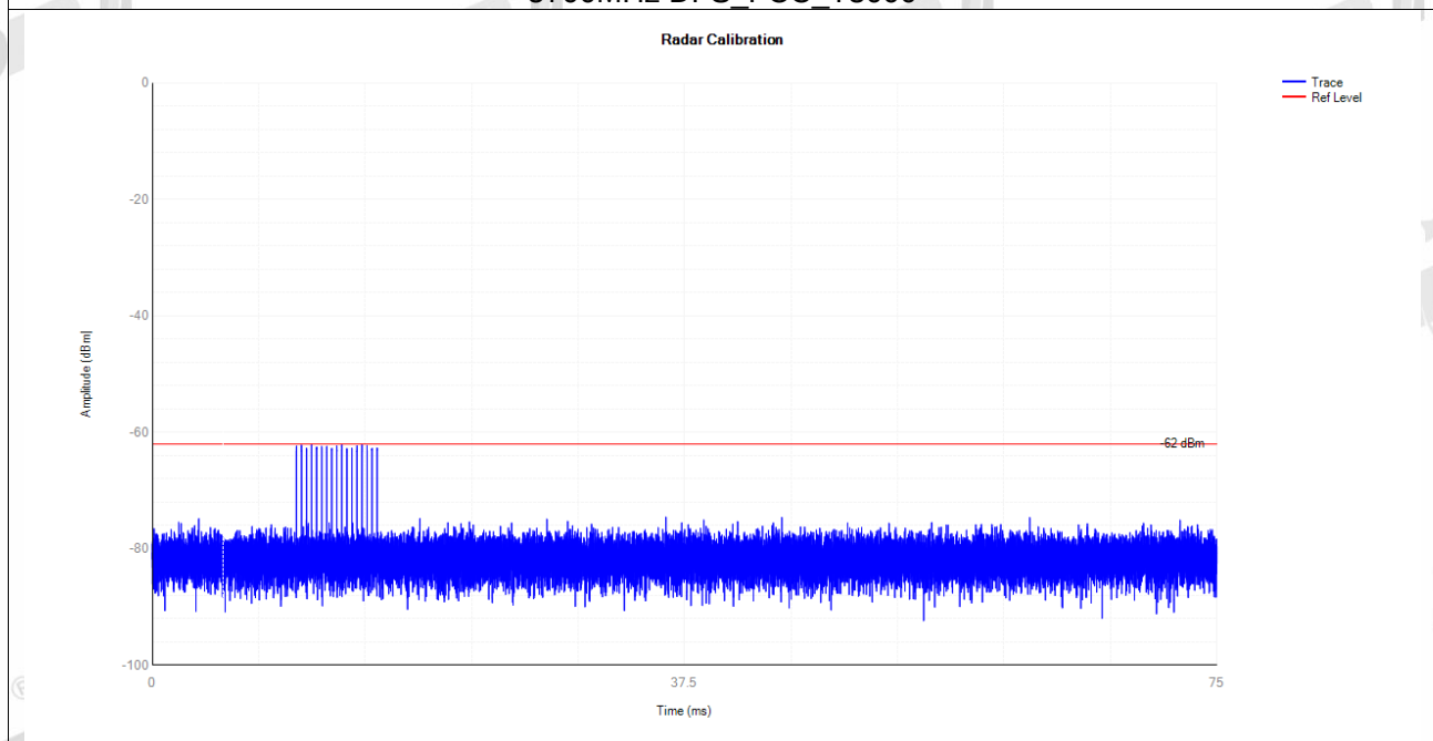
5700MHz DFS_FCC_T4000
