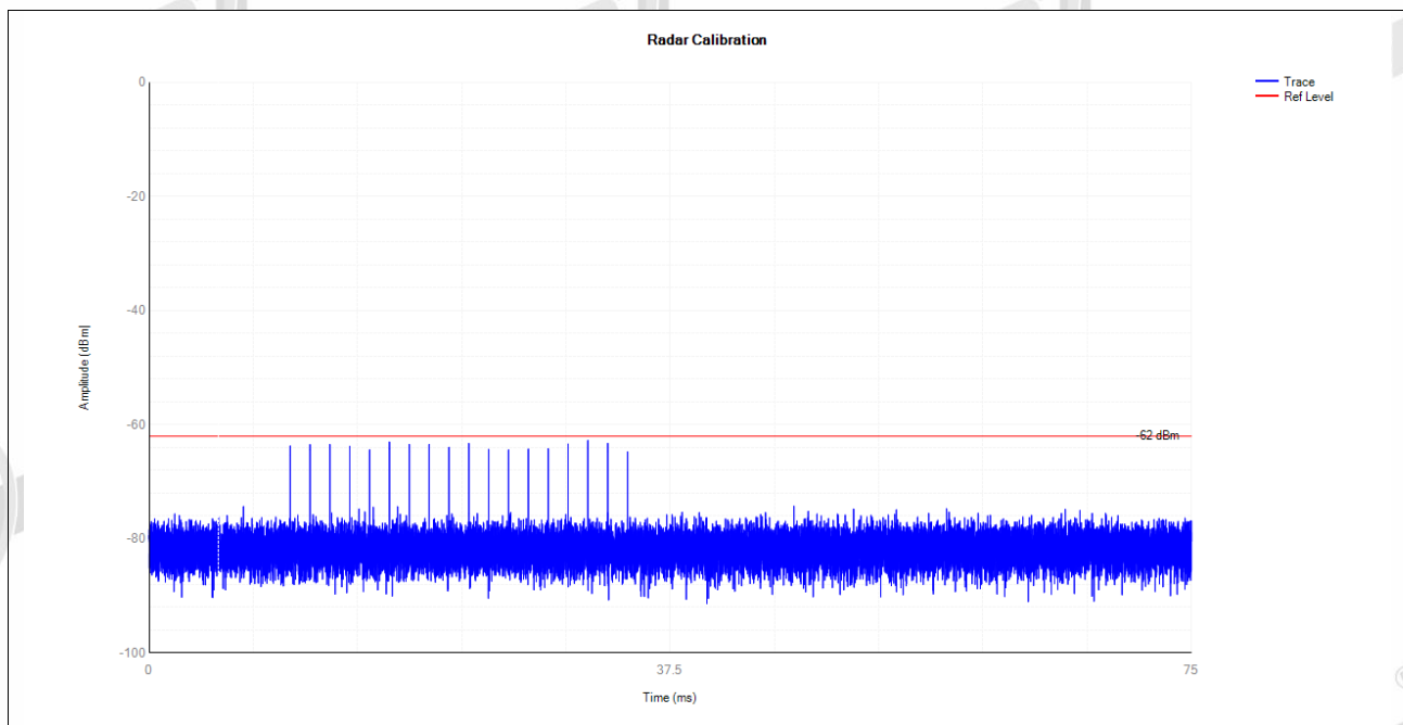
5700MHz DFS_FCC_T1000
