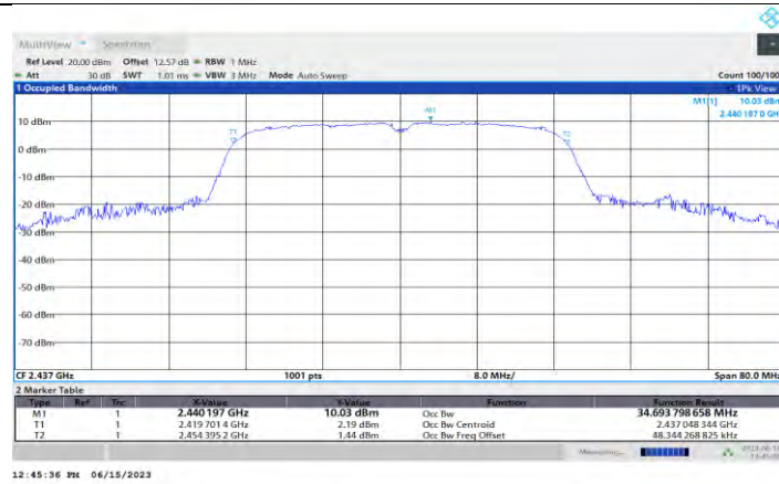
11N40SISO_Ant1_2437
