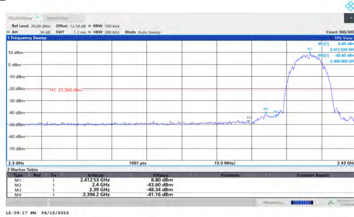
11B_Ant1_Low_2412
