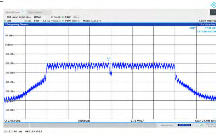
11G_Ant1_2412
