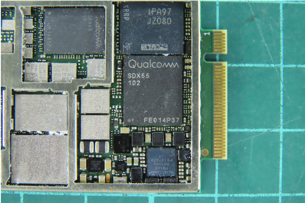
(19) EUT Photo
