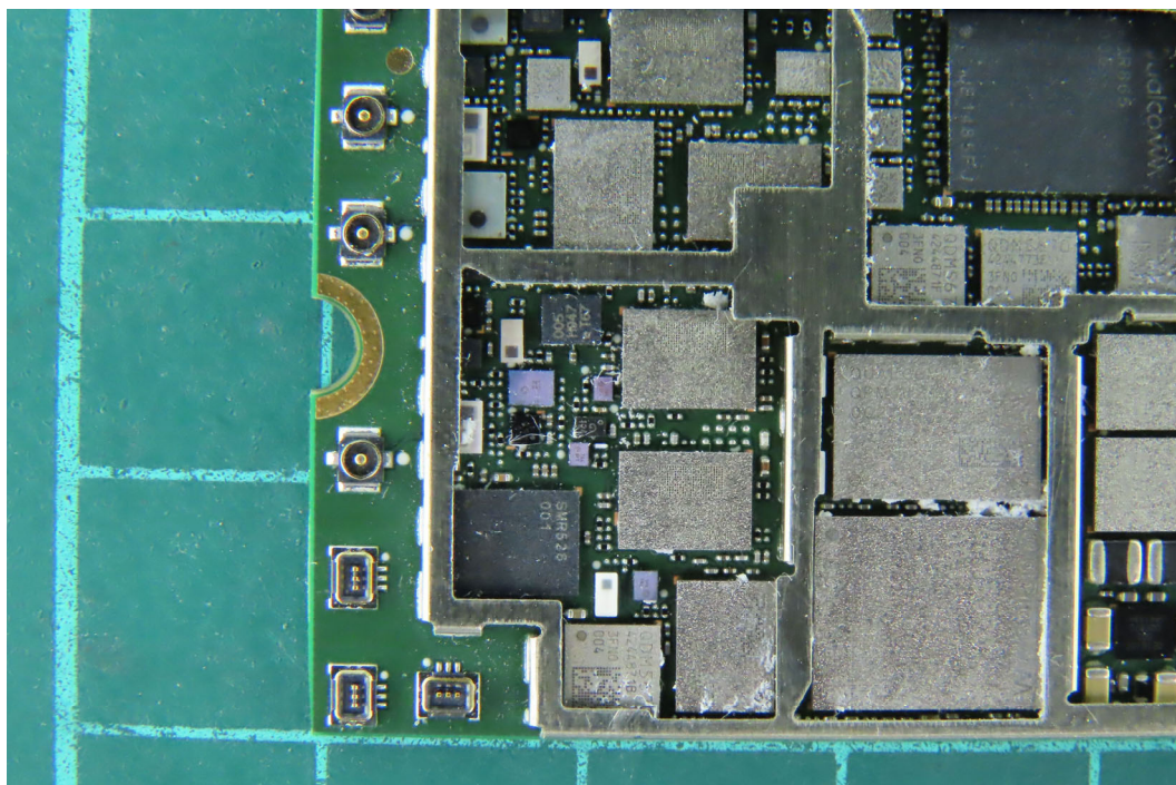
(18) EUT Photo
