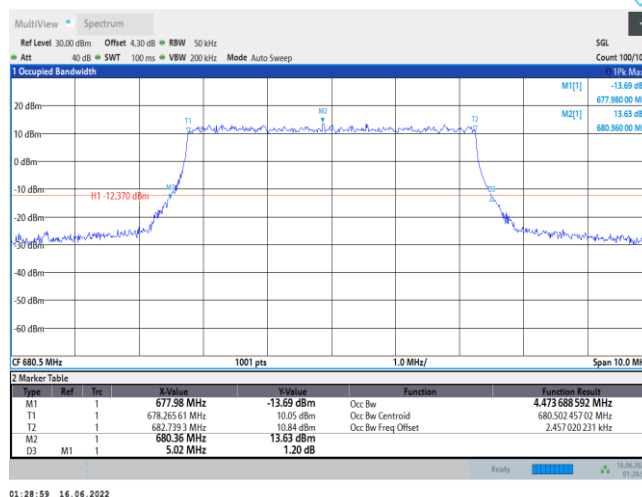
Band71-5MHz-QPSK-133297-25RB#0
