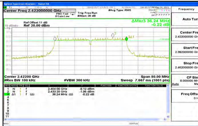
11N40SISO Ant1 2422
