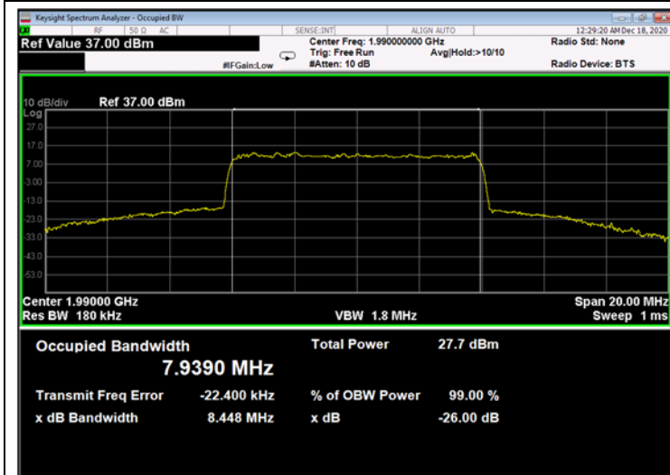
Figure 749: QPSK 10MHz B.W.; 1990.0MHz, 60kHz - Output
