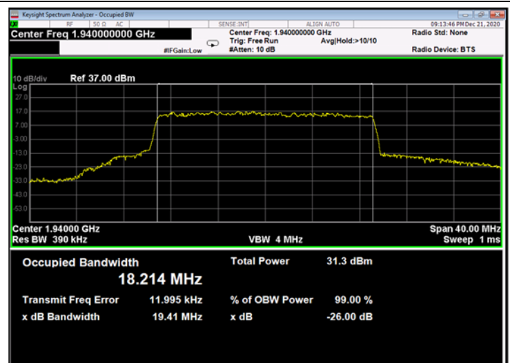
Figure 694: 256QAM 20MHz B.W.; 1940.0MHz, 30kHz - Output
