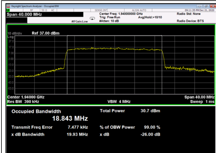
Figure 693: 256QAM 20MHz B.W.; 1940.0MHz, 15kHz - Output
