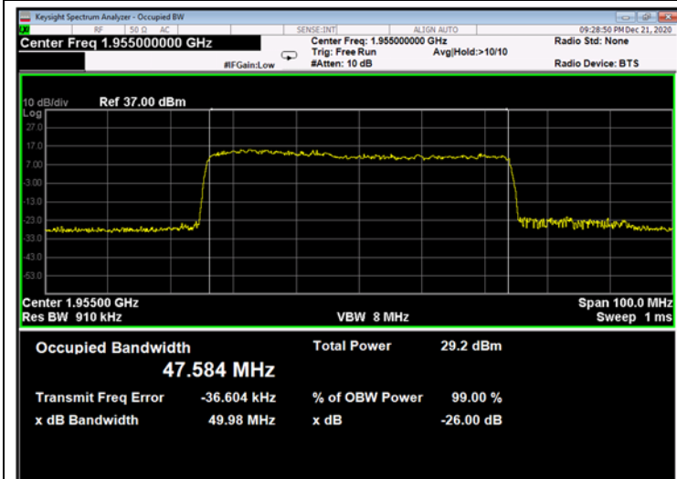
Figure 721: 256QAM 50MHz B.W.; 1955.0MHz, 30kHz - Output
