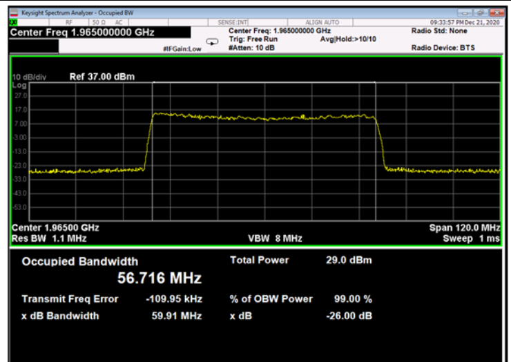
Figure 734: 256QAM 60MHz B.W.; 1965.0MHz, 60kHz - Output
