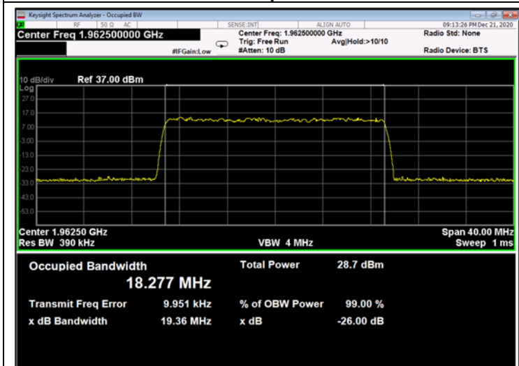
Figure 697: 256QAM 20MHz B.W.; 1962.5MHz, 30kHz - Output
