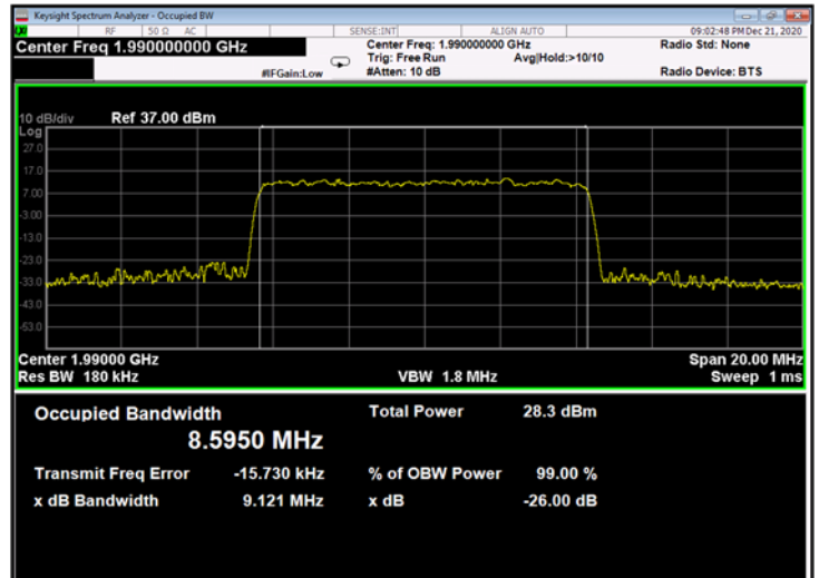
Figure 682: 256QAM 10MHz B.W.; 1990.0MHz, 30kHz - Output
