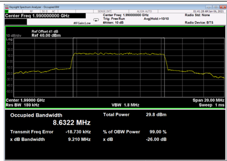
Figure 748: QPSK 10MHz B.W.; 1990.0MHz, 30kHz - Output
