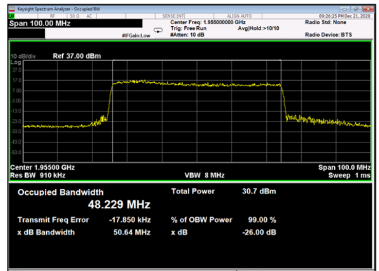
Figure 720: 256QAM 50MHz B.W.; 1955.0MHz, 15kHz - Output
