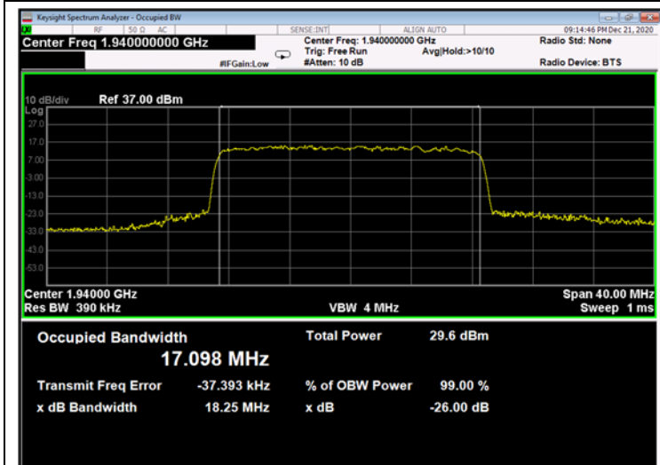
Figure 695: 256QAM 20MHz B.W.; 1940.0MHz, 60kHz - Output
