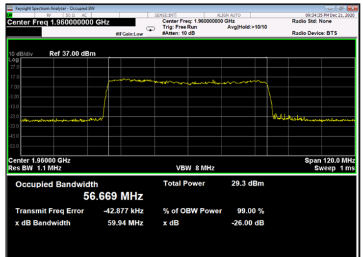
Figure 730: 256QAM 60MHz B.W.; 1960.0MHz, 60kHz - Output
