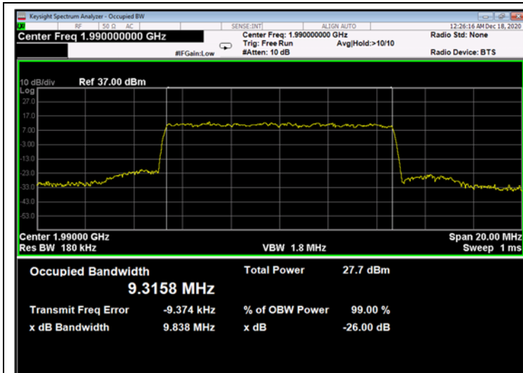
Figure 747: QPSK 10MHz B.W.; 1990.0MHz, 15kHz - Output
