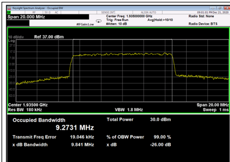
Figure 675: 256QAM 10MHz B.W.; 1935.00MHz, 15kHz - Output
