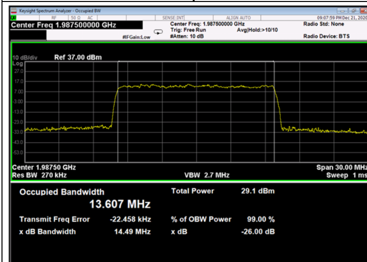
Figure 691: 256QAM 15MHz B.W.; 1987.5MHz, 30kHz - Output
