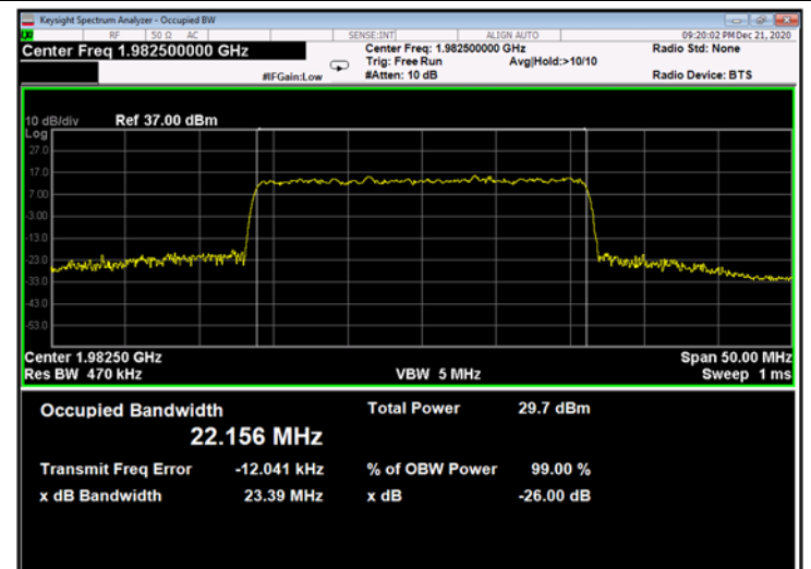
Figure 710: 256QAM 25MHz B.W.; 1982.5MHz, 60kHz - Output
