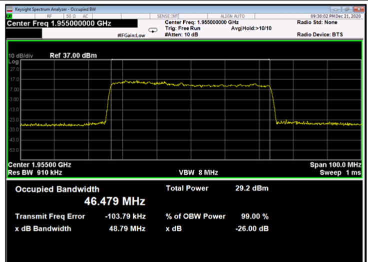
Figure 722: 64QAM 50MHz B.W.; 1955.0MHz, 60kHz - Output
