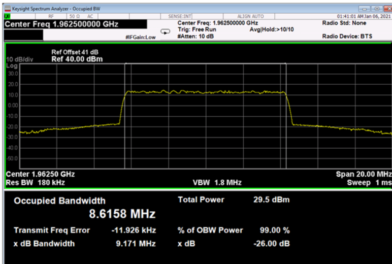
Figure 745: QPSK 10MHz B.W.; 1962.5MHz, 30kHz - Output
