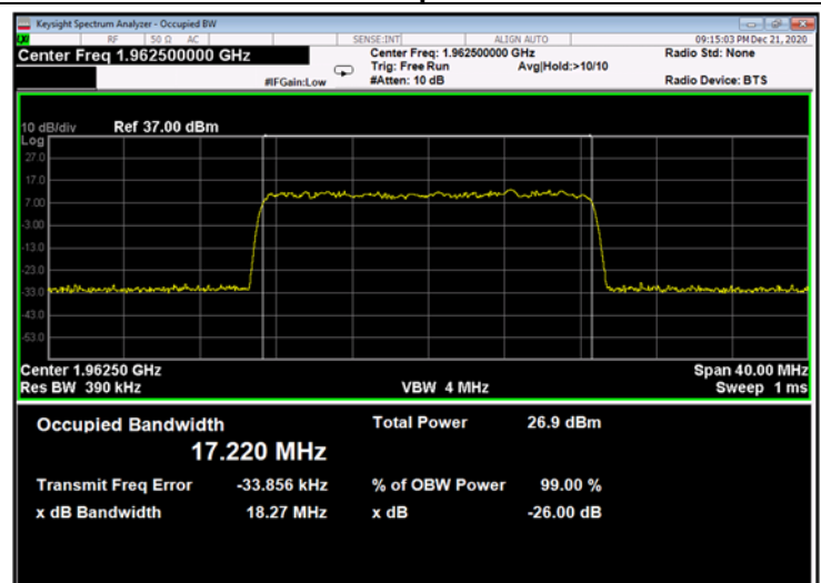
Figure 698: 256QAM 20MHz B.W.; 1962.5MHz, 60kHz - Output
