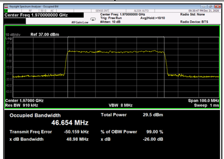
Figure 728: 256QAM 50MHz B.W.; 1970.0MHz, 60kHz - Output
