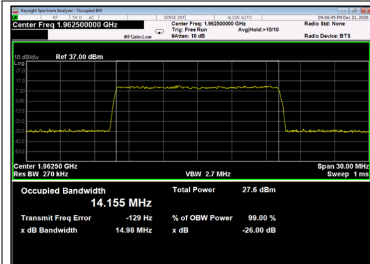
Figure 687: 256QAM 15MHz B.W.; 1962.5MHz, 15kHz - Output
