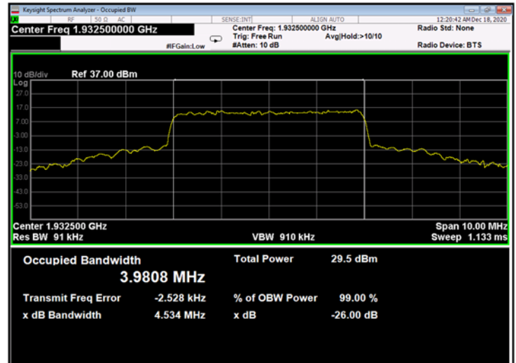
Figure 736: QPSK 5MHz B.W.; 1932.5MHz, 30kHz - Output
