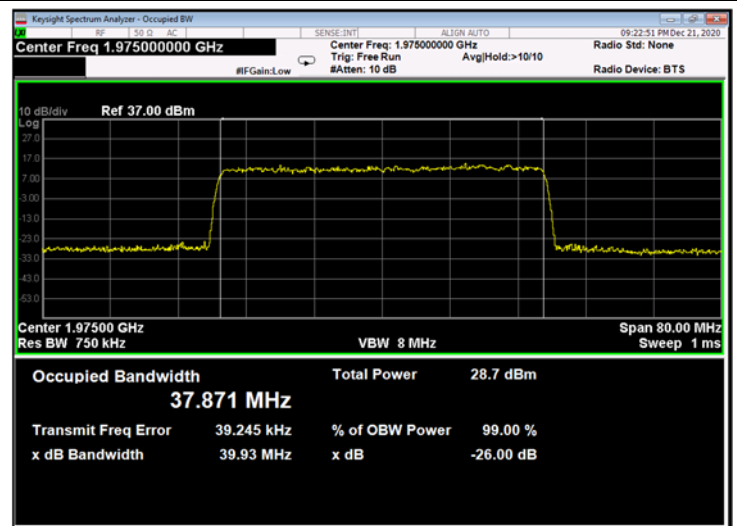
Figure 718: 256QAM 40MHz B.W.; 1975.0MHz, 30kHz - Output
