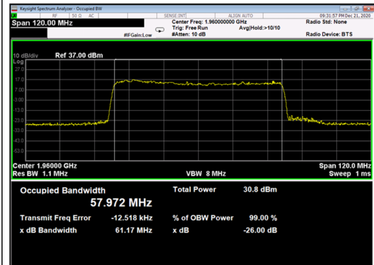
Figure 729: 256QAM 60MHz B.W.; 1960.0MHz, 30kHz - Output
