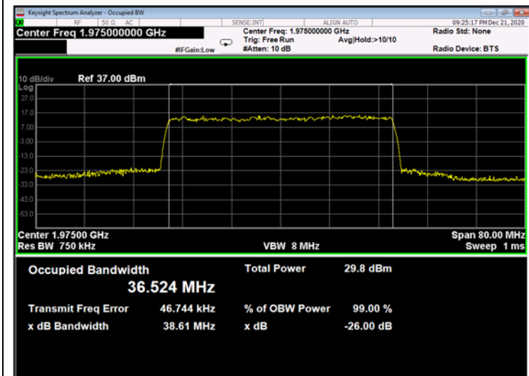
Figure 719: 256QAM 40MHz B.W.; 1975.0MHz, 60kHz - Output
