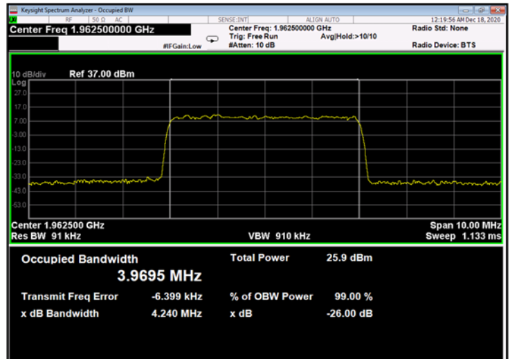
Figure 738: QPSK 5MHz B.W.; 1962.5MHz, 30kHz - Output
