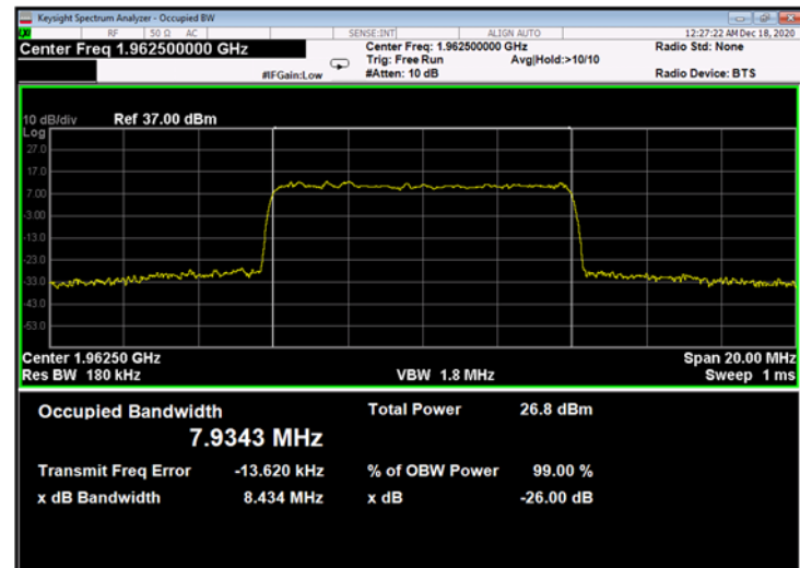
Figure 746: QPSK 10MHz B.W.; 1962.5MHz, 60kHz - Output
