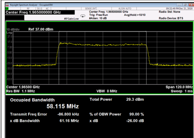
Figure 733: 256QAM 60MHz B.W.; 1965.0MHz, 30kHz - Output
