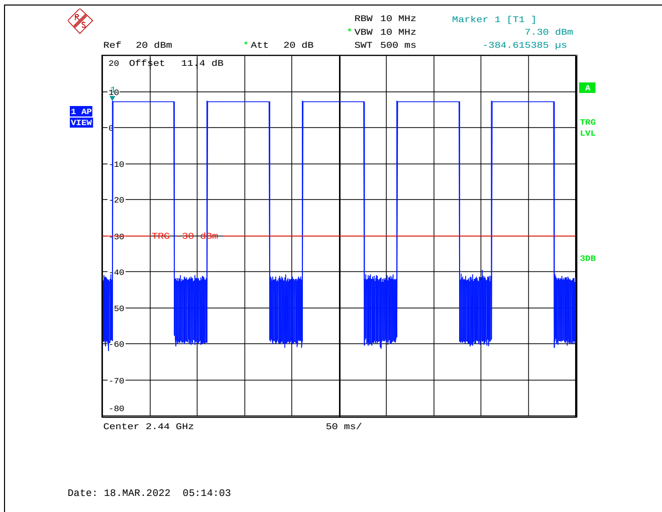
Plot 5.7.4.1.1. Duty Cycle (Pulse Train)
