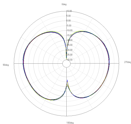
YZ-plane
