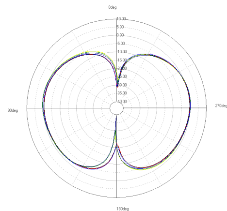
ZX-plane
