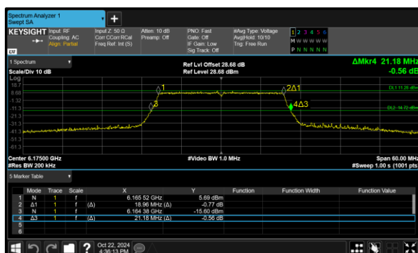
Figure 163 - 802.11ax HE20 SU SP Minimum 26 dB EBW
