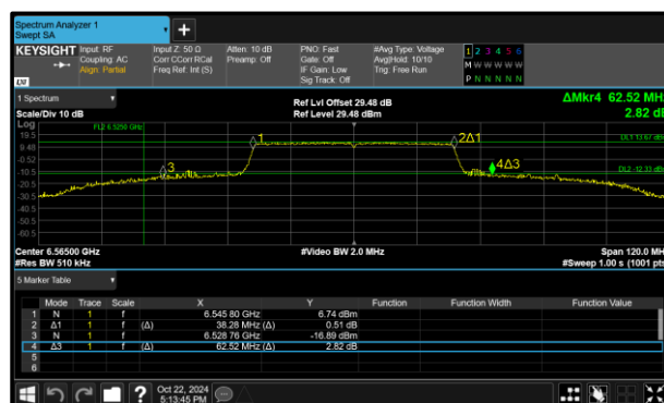
Figure 166 - 802.11ax HE40 SU SP Maximum 26 dB EBW
