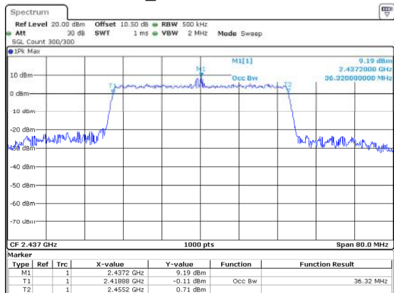
802.11n40_2437MHz 36.320MHz
