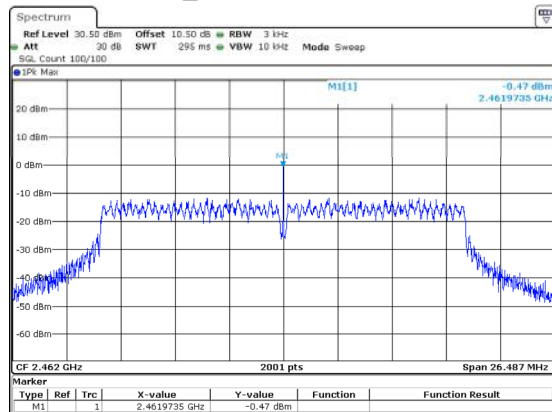
802.11n20_2462MHz -0.47dBm/3kHz
