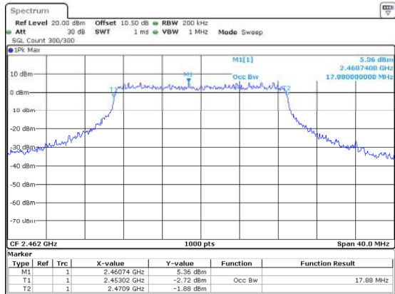
802.11n20_2462MHz 17.880MHz
