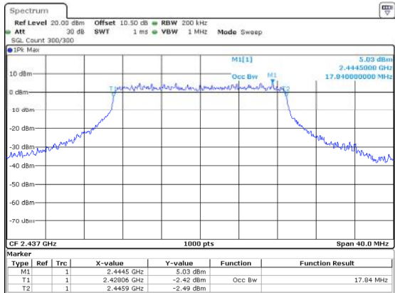
802.11n20_2437MHz 17.840MHz
