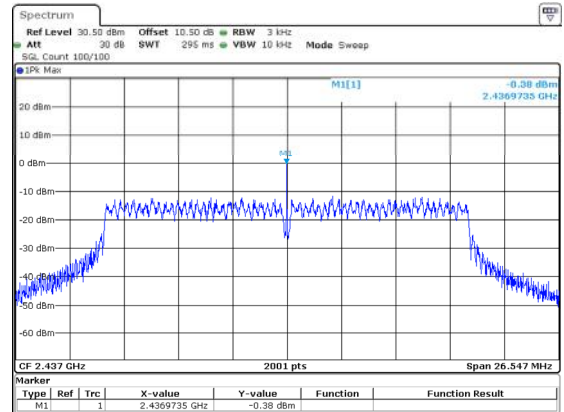
802.11n20_2437MHz -0.38dBm/3kHz
