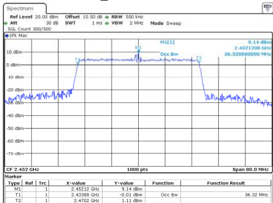
802.11n40_2452MHz 36.320MHz
