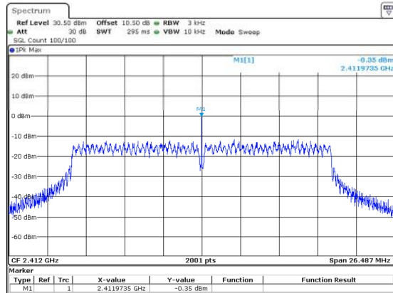
802.11n20_2412MHz -0.35dBm/3kHz
