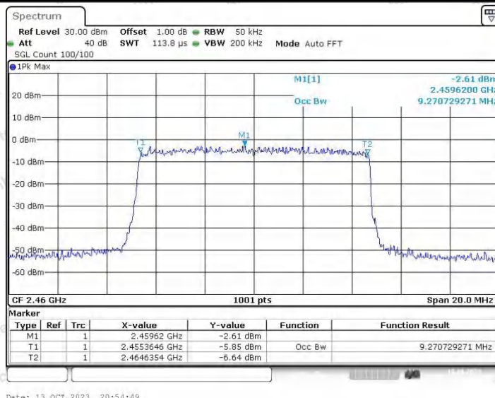
10M_Ant2_2460
