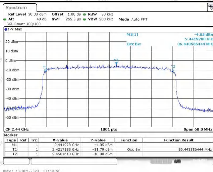
40M_Ant2_2440
