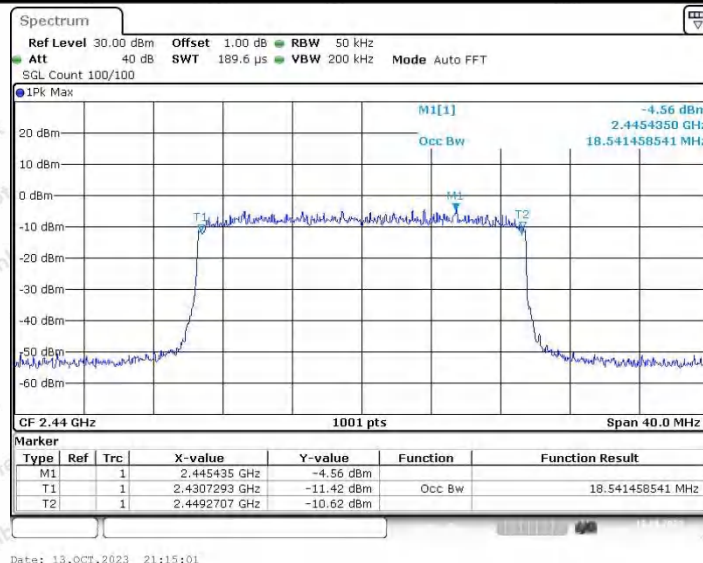
20M_Ant2_2440
