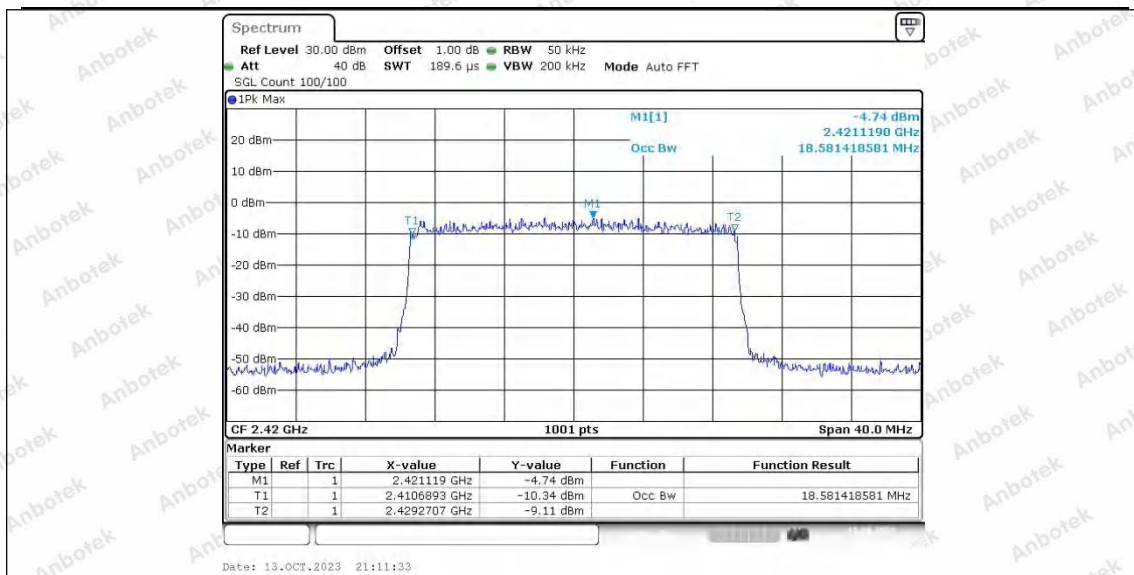
20M_Ant2_2420
