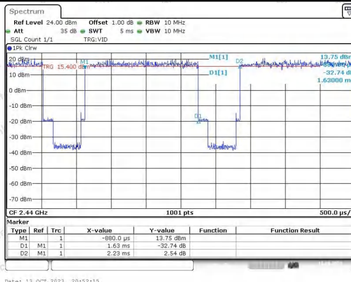
10M_Ant2_2440
