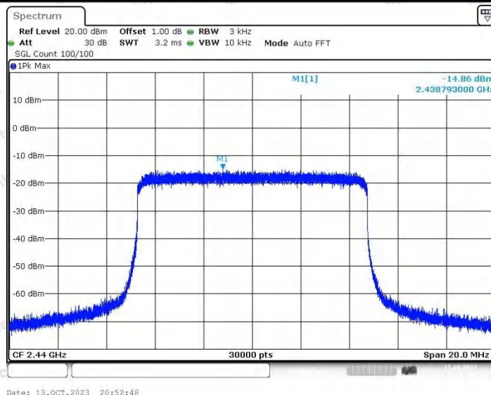
10M_Ant2_2440
