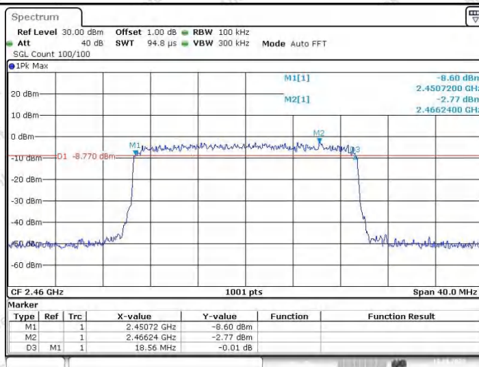
20M_Ant2_2460
