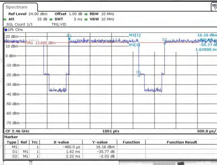
20M_Ant2_2460
