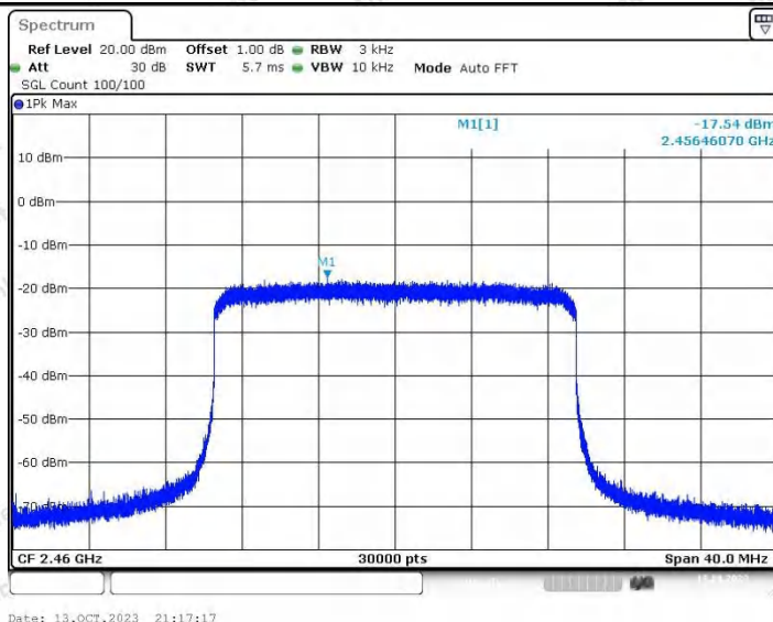
20M_Ant2_2460
