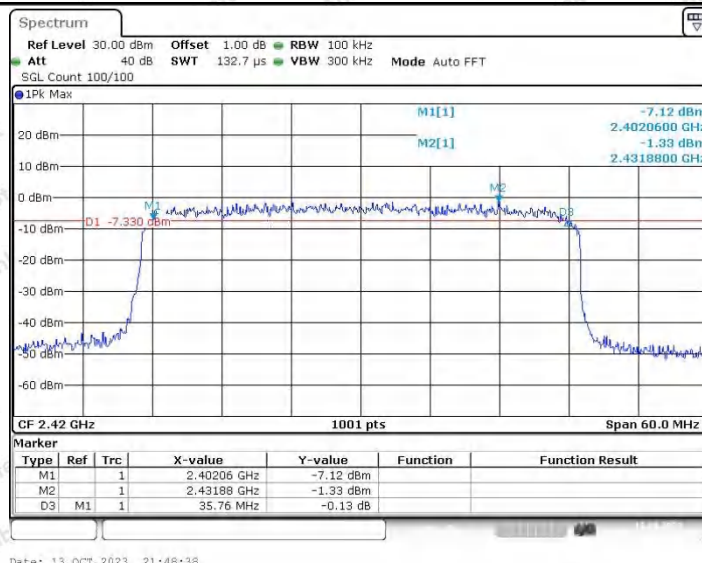
40M_Ant2_2420
