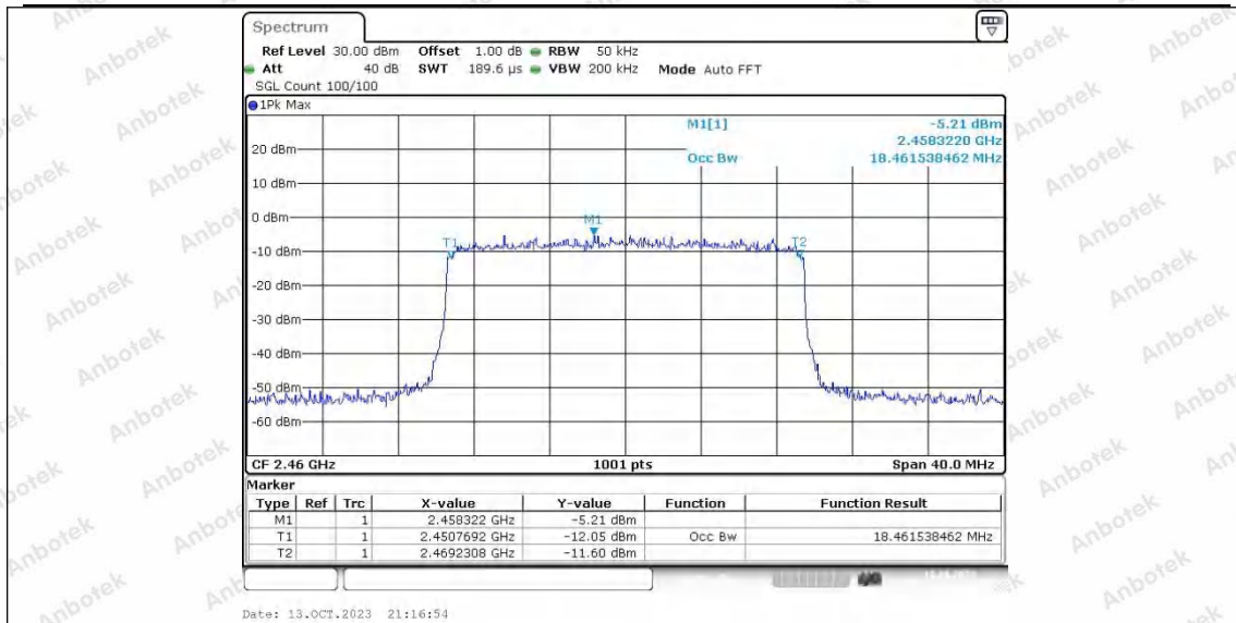
20M_Ant2_2460
