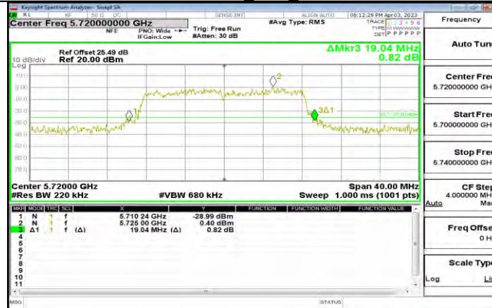
11A-CDD Ant9 5720
