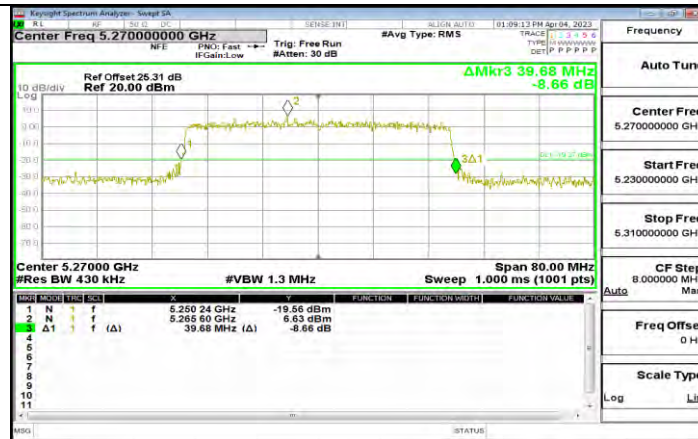
11AX40MIMO Ant9 5270
