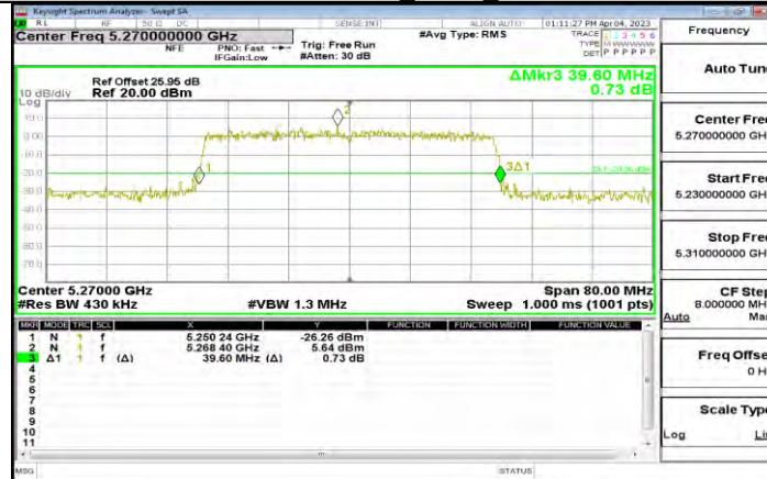
11AX40MIMO Ant15 5270
