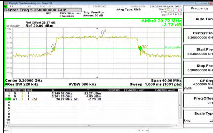
11AX20MIMO_Ant3_5260
