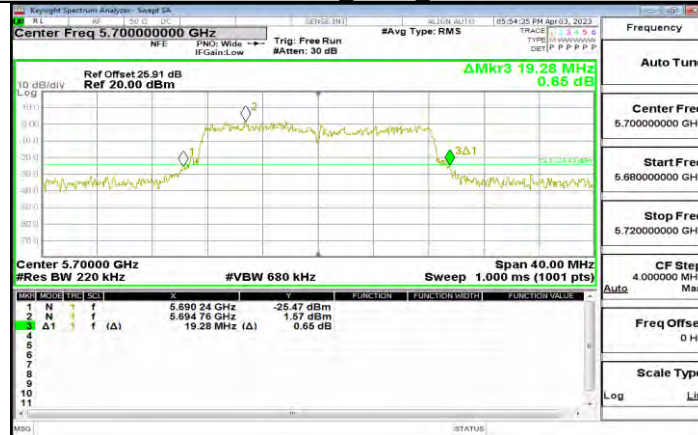
11A-CDD Ant15 5700
