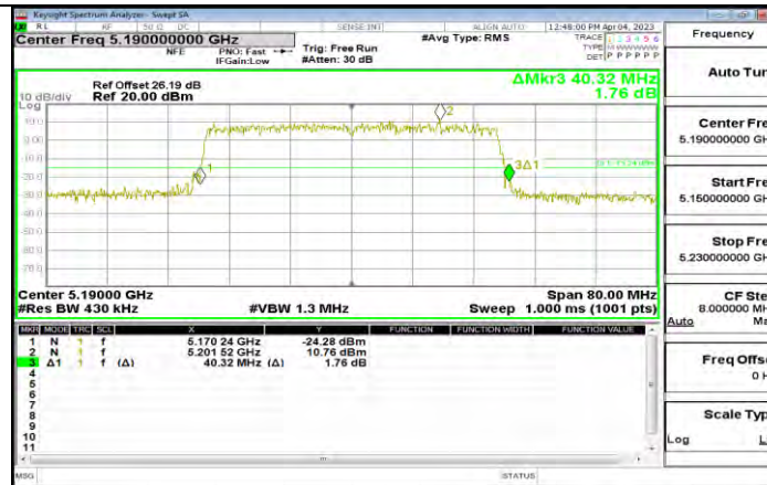
11AX40MIMO Ant10 5190
