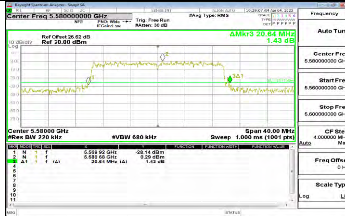
11AX20MIMO_Ant2_5580
