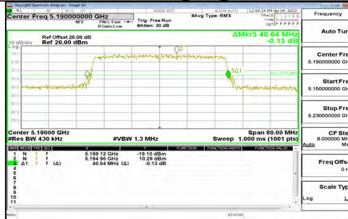
11AX40MIMO Ant15 5190
