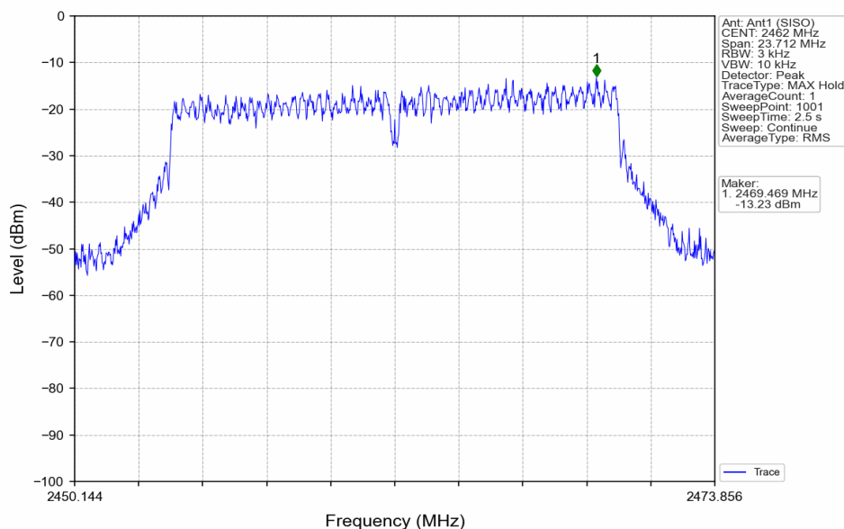
802.11g_HCH_2462MHz_Ant1 (SISO)_NTNV
