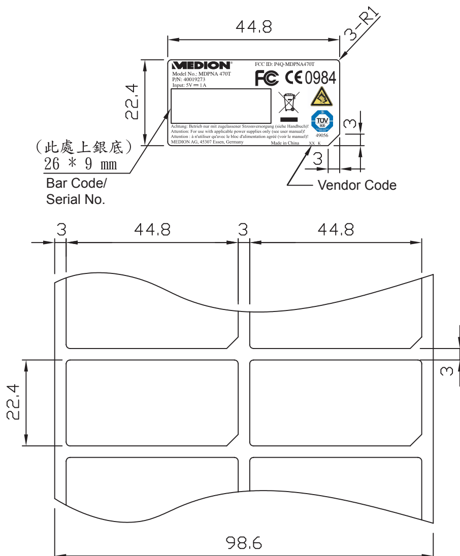
< 刀模圖 > 1:1
