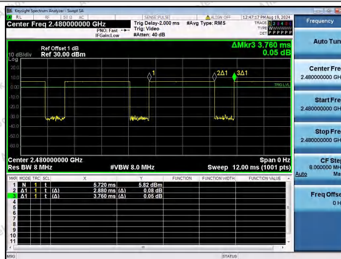
NTNV-DH5-Ant1-2480
