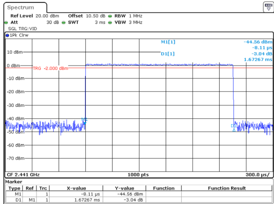
DH3_Hopping 1.673ms
