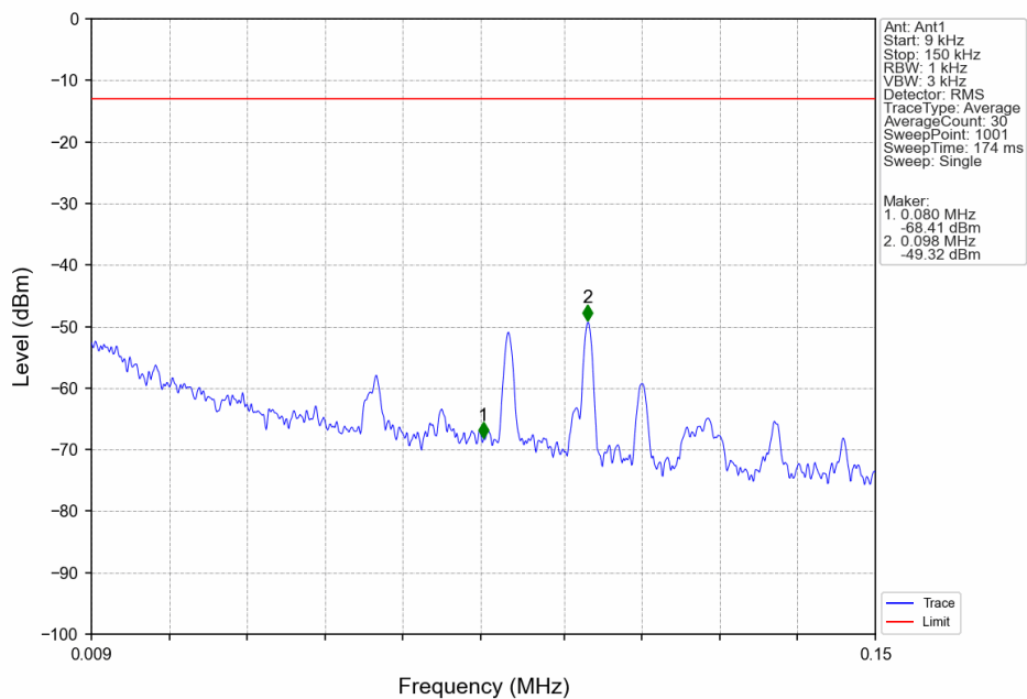
Band4 1.4MHz 16QAM LCH 1710.7MHz RB 1 0 NTV
