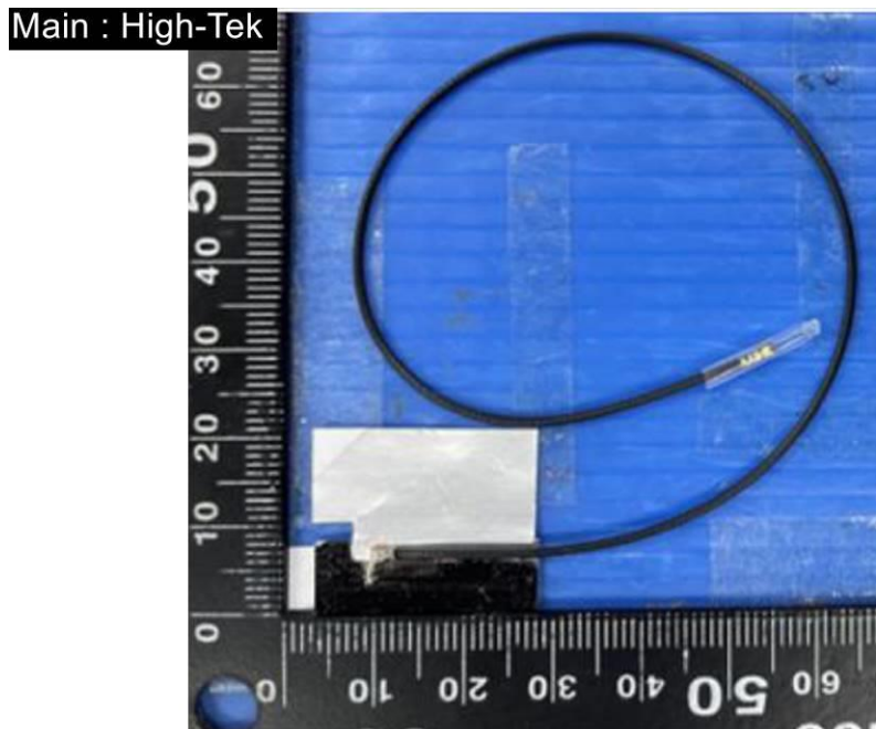
EUT Photo (12)
