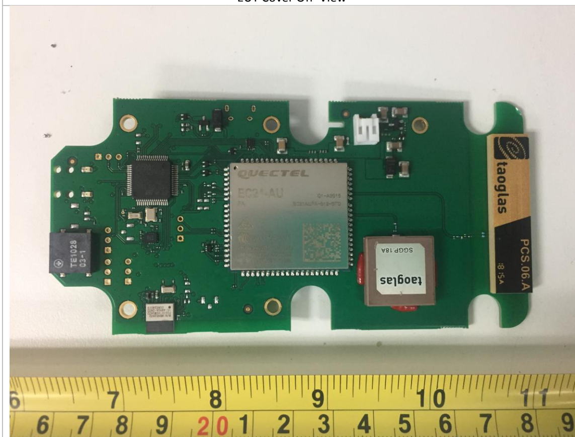
EUT Main PCBA - Top
