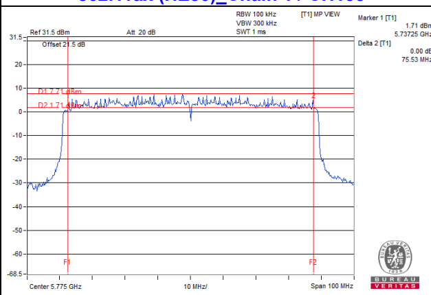
802.11ax (HE80)_Chain 1 / CH155
