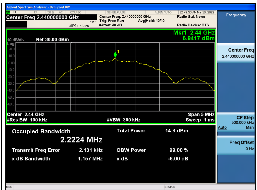
Test_Graph_O-QPSK_ANT1_2440_DTSBW
