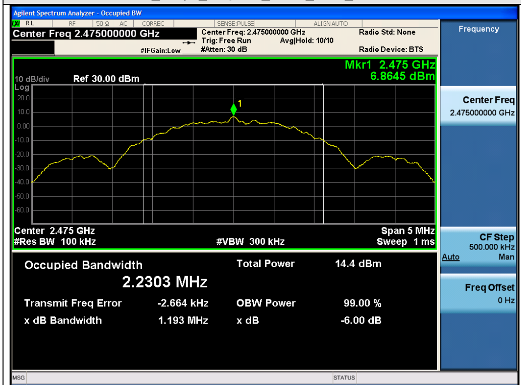
Test_Graph_O-QPSK_ANT1_2475_DTSBW
