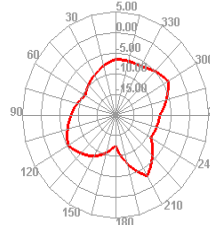
2500.000MHz E1
