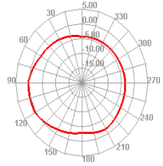
2400.000MHz E2
