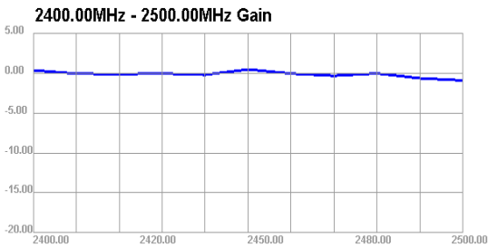
2450.000MHz E2
