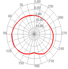
2450.000MHz H
