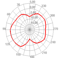
2450.000MHz H
