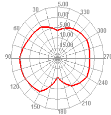
2500.000MHz H
