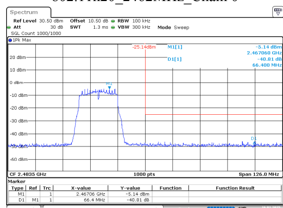
802.11n20_2462MHz_Chain 0
