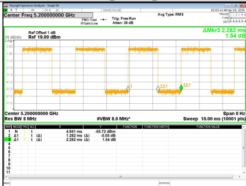
IEEE 802.11ac_20MHz_Channel 40
