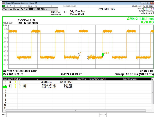
IEEE 802.11ac_40MHz_Channel 38
