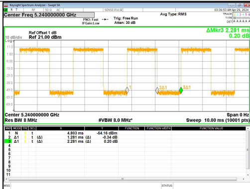
IEEE 802.11ac_20MHz_Channel 48
