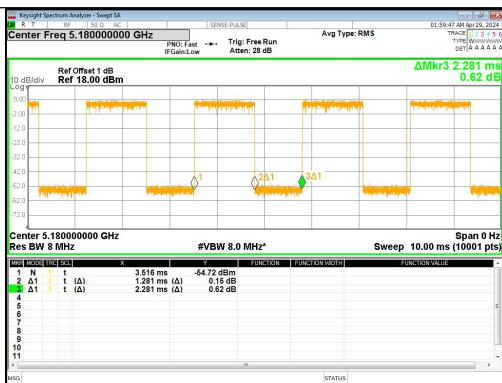
IEEE 802.11ac_20MHz_Channel 36
