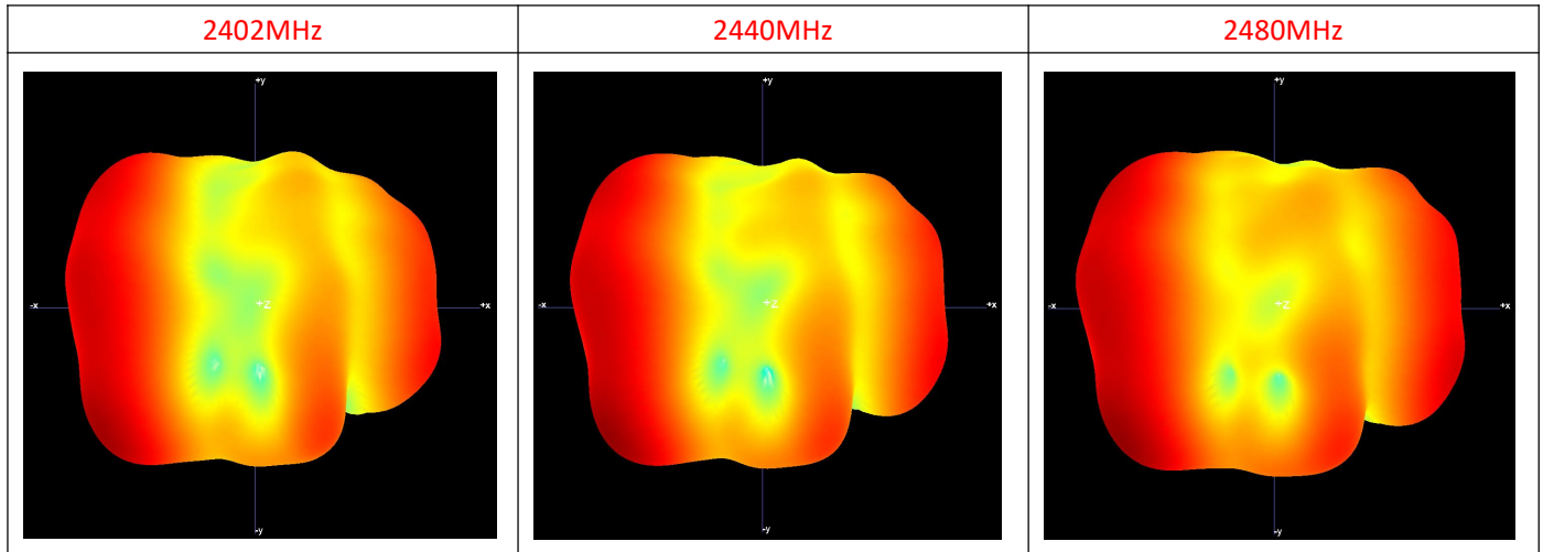
3D 方向图
