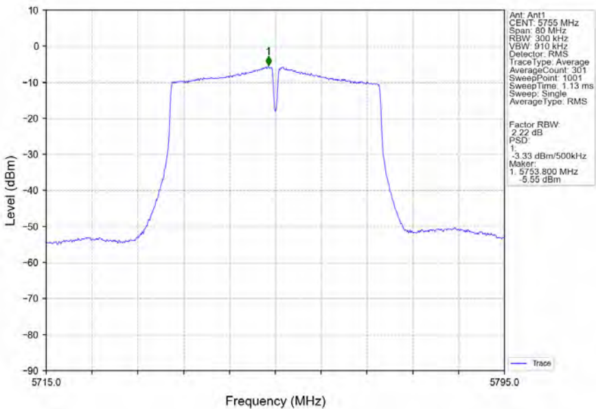
802.11n(HT40)_LCH_5755MHz_Ant1_NTNV
