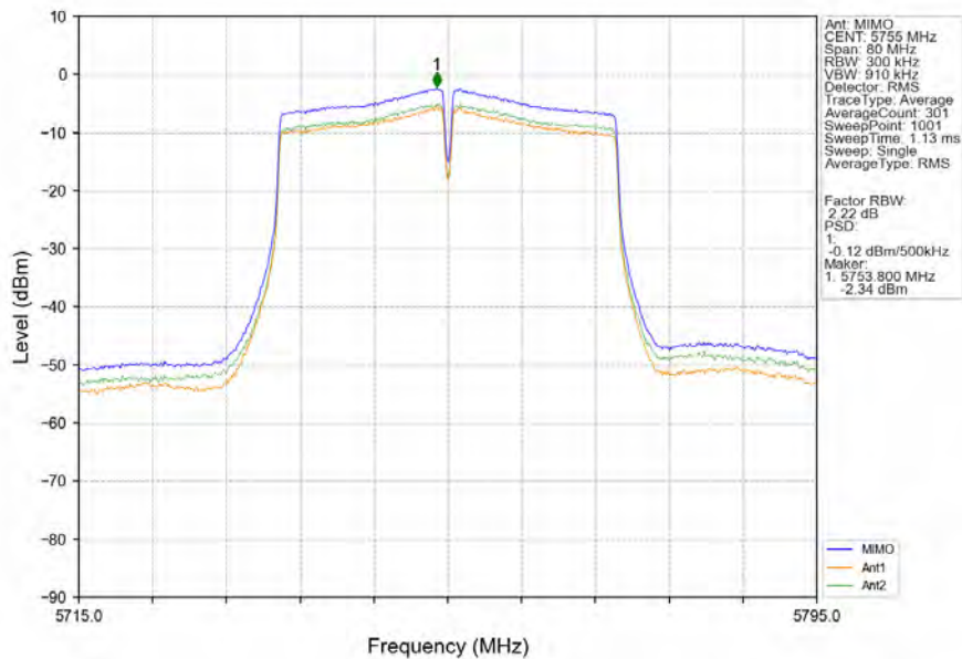
802.11n(HT40)_LCH_5755MHz_MIMO_NTNV
