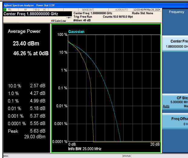
Band2-10MHz-QPSK-18900-1RB#0-PASS
