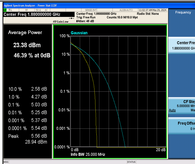
Band2-3MHz-QPSK-18900-1RB#0-PASS
