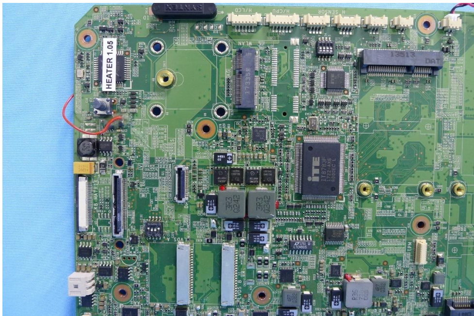
(13) EUT Photo
