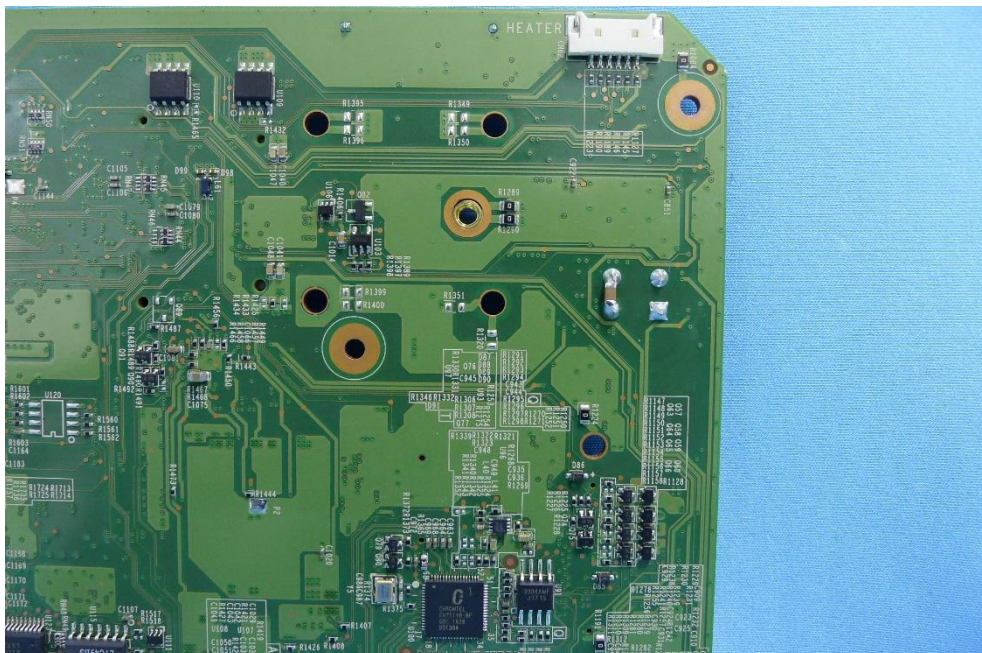
(21) EUT Photo
