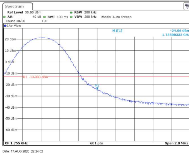
Band4-10MHz-QPSK-20350-1RB#0
