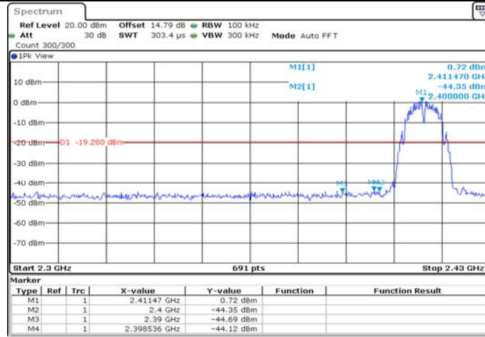
11B_Ant1_Low_2412
