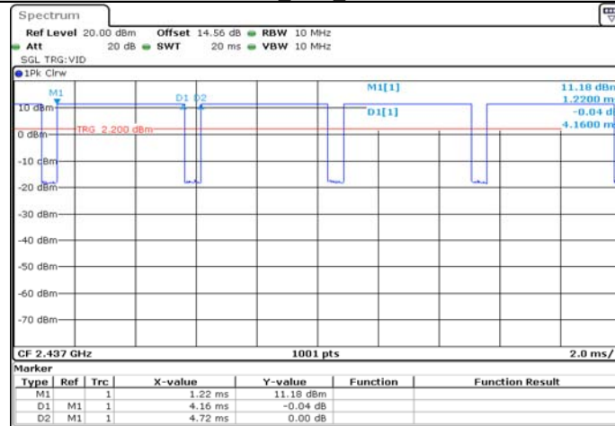
11B_Ant1_2437
