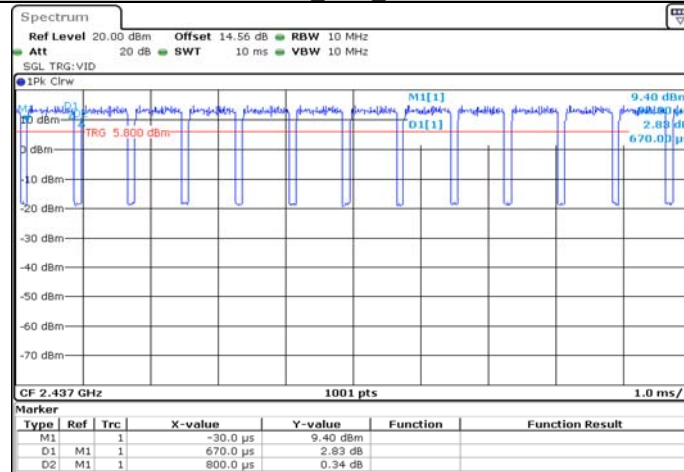
11G_Ant1_2437
