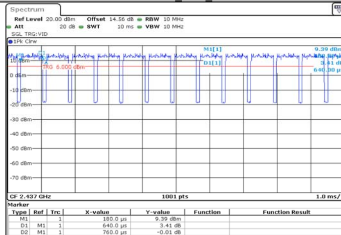
11N20SISO_Ant1_2437
