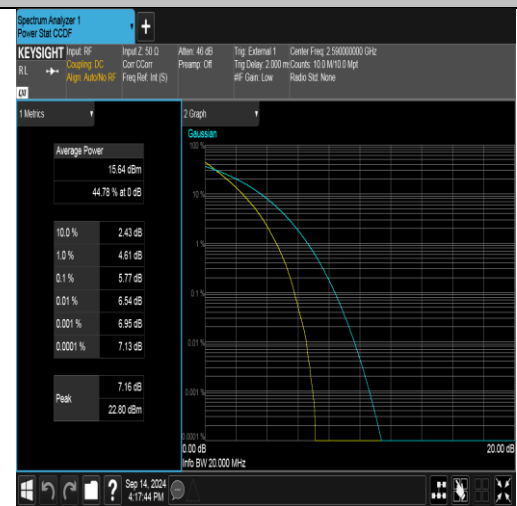
Band41(2535-2655)-20MHz-QPSK-40590-100RB#0-PASS
