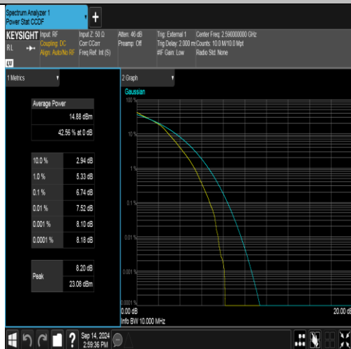
Band41(2535-2655)-10MHz-16QAM-40590-50RB#0-PASS
