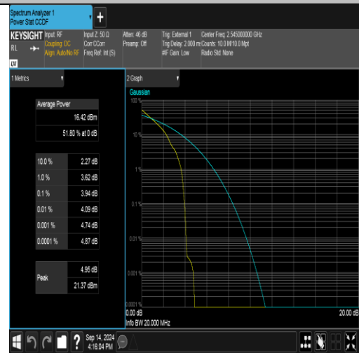
Band41(2535-2655)-20MHz-QPSK-40140-1RB#0-PASS
