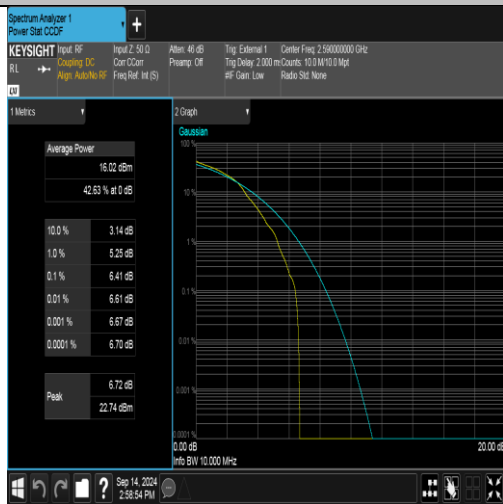
Band41(2535-2655)-10MHz-16QAM-40590-1RB#0-PASS
