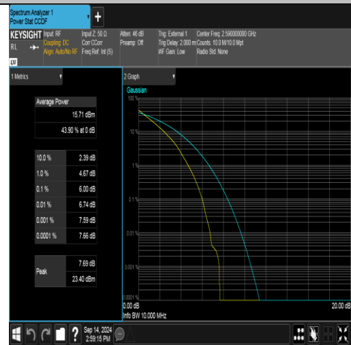
Band41(2535-2655)-10MHz-QPSK-40590-50RB#0-PASS
