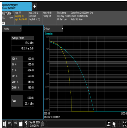
Band41(2535-2655)-10MHz-16QAM-41190-1RB#0-PASS
