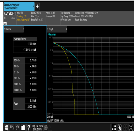
Band41(2535-2655)-10MHz-QPSK-41190-1RB#0-PASS
