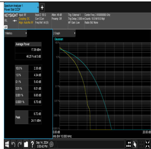
Band41(2535-2655)-10MHz-QPSK-41190-50RB#0-PASS
