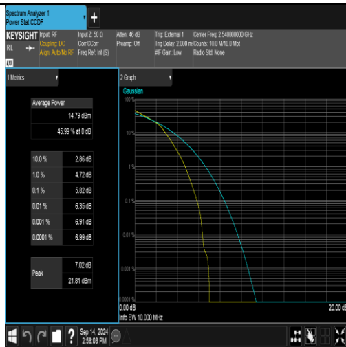
Band41(2535-2655)-10MHz-16QAM-40090-50RB#0-PASS
