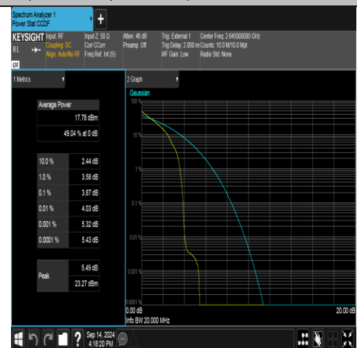
Band41(2535-2655)-20MHz-QPSK-41140-1RB#0-PASS
