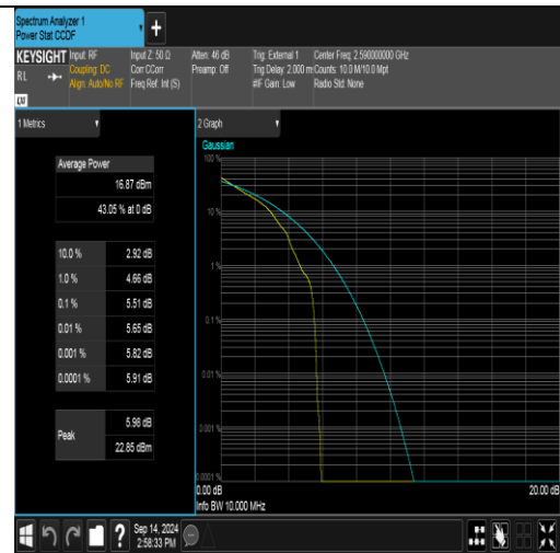
Band41(2535-2655)-10MHz-QPSK-40590-1RB#0-PASS
