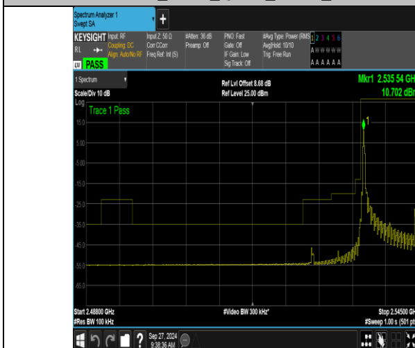
Band41_10MHz_QPSK_40090_1RB#0
