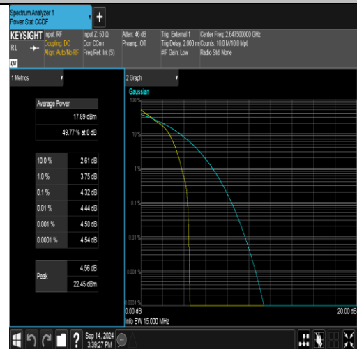
Band41(2535-2655)-15MHz-QPSK-41165-1RB#0-PASS
