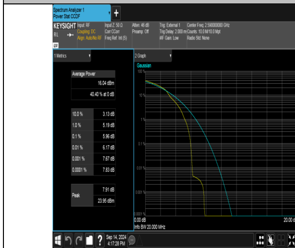
Band41(2535-2655)-20MHz-16QAM-40590-1RB#0-PASS
