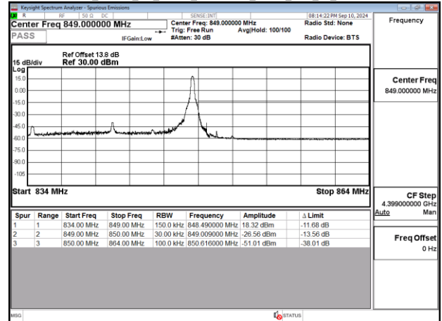
Band5_15MHz_CP_OFDM_SCS15kHz_QPSK_RB1_78_CH168300
