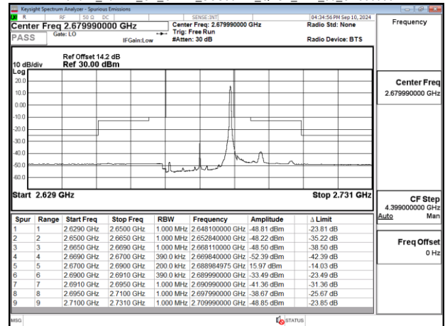
Band41 20MHz CP OFDM_SCS30kHz QPSK RB1_50_CH535998
