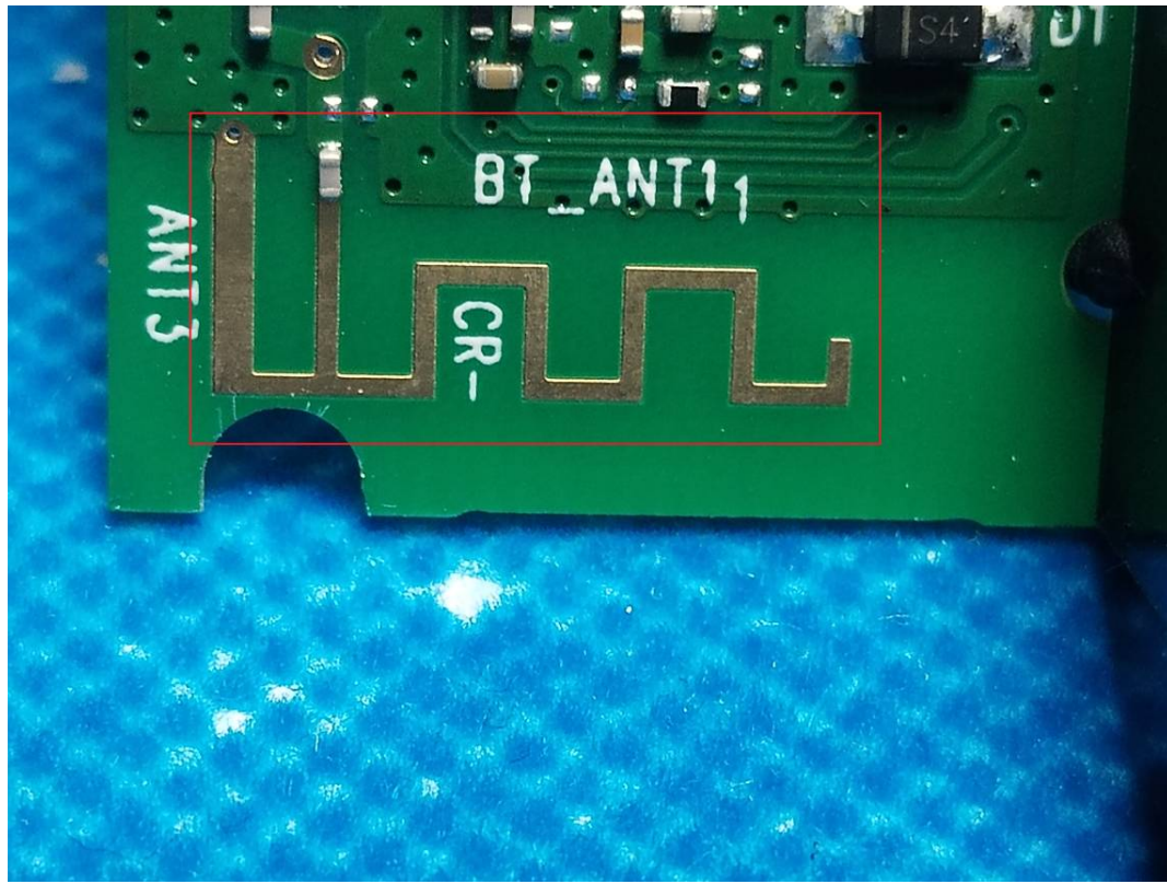
BT ANT
