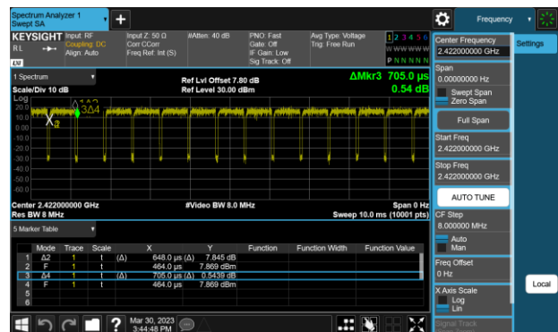
802.11ax HE40
