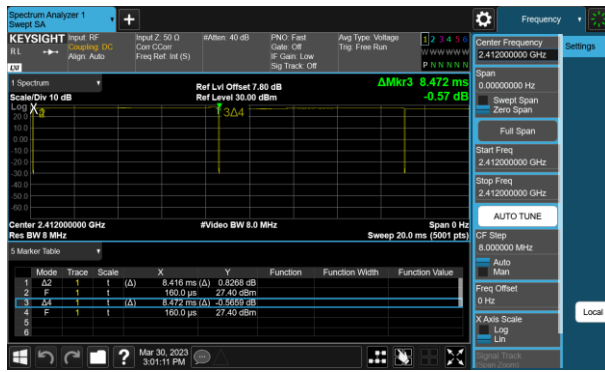
802.11n HT20
