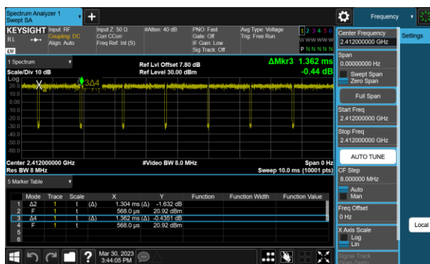
802.11ax HE20
