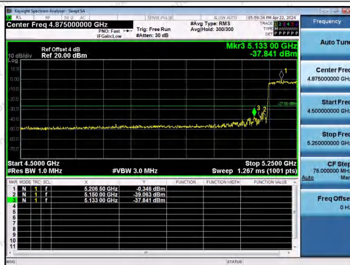
11AX80MIMO-Ant1-5210-PASS
