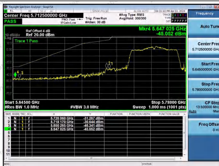
11N40MIMO-Ant1-5755-PASS
