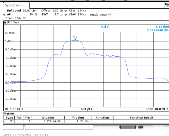
11AX20MIMO_Ant3_5580_52Tone_RU38
