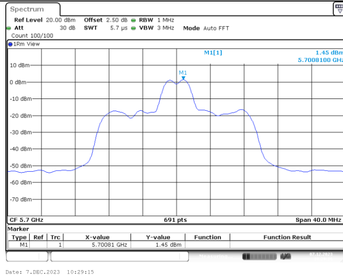
11AX20MIMO_Ant1_5700_26Tone_RU4
