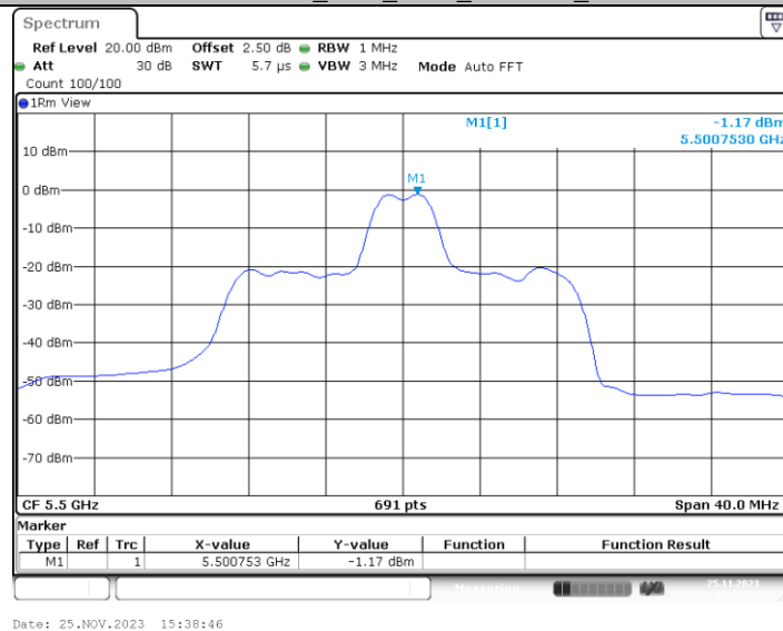
11AX20MIMO_Ant2_5500_26Tone_RU4
