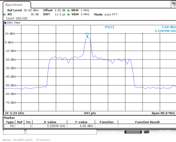
11AX40MIMO_Ant1_5230_26Tone_RU8
