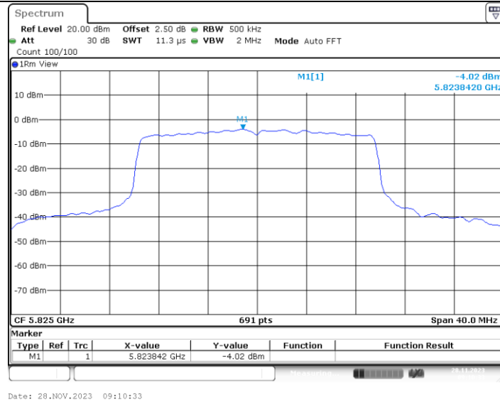
11AX20MIMO_Ant1_5825_242Tone_RU61
