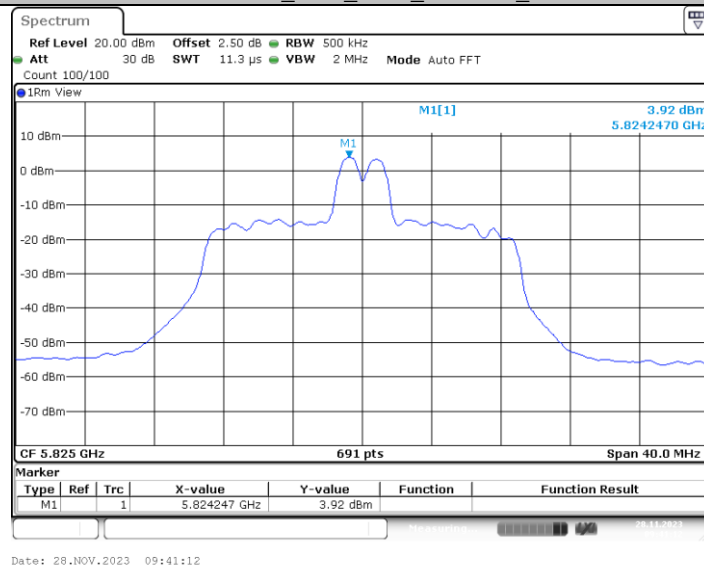
11AX20MIMO_Ant2_5825_26Tone_RU4
