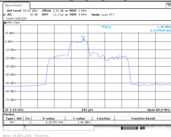
11AX40MIMO_Ant1_5230_106Tone_RU54
