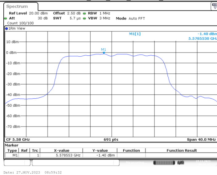
11AX20MIMO_Ant1_5580_242Tone_RU61
