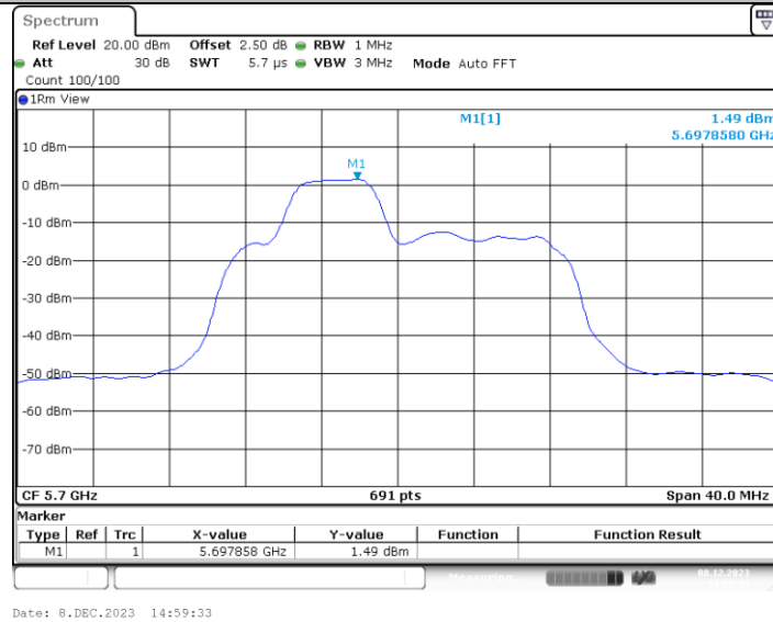
11AX20MIMO_Ant1_5700_52Tone_RU38
