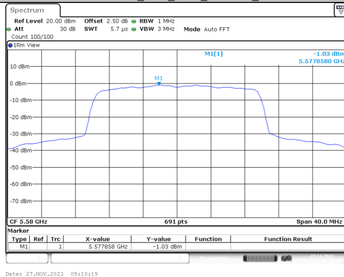
11AX20MIMO_Ant3_5580_242Tone_RU61
