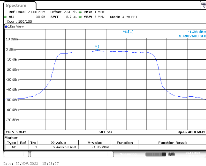
11AX20MIMO_Ant1_5500_242Tone_RU61
