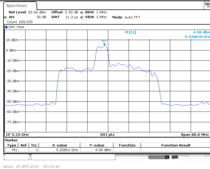
11AX40MIMO_Ant1_5230_52Tone_RU40
