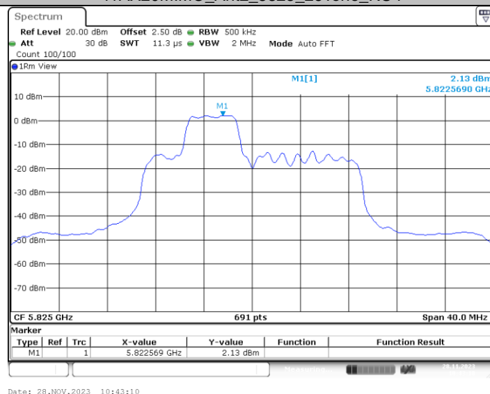
11AX20MIMO_Ant2_5825_52Tone_RU38
