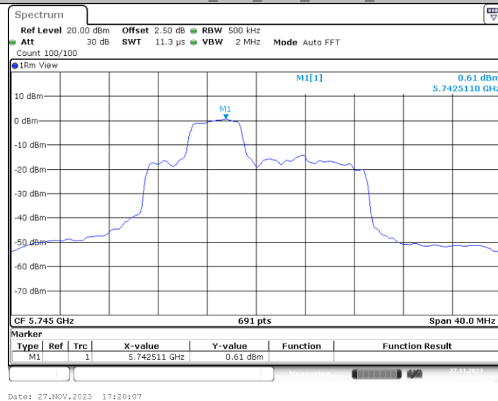
11AX20MIMO_Ant3_5745_52Tone_RU38
