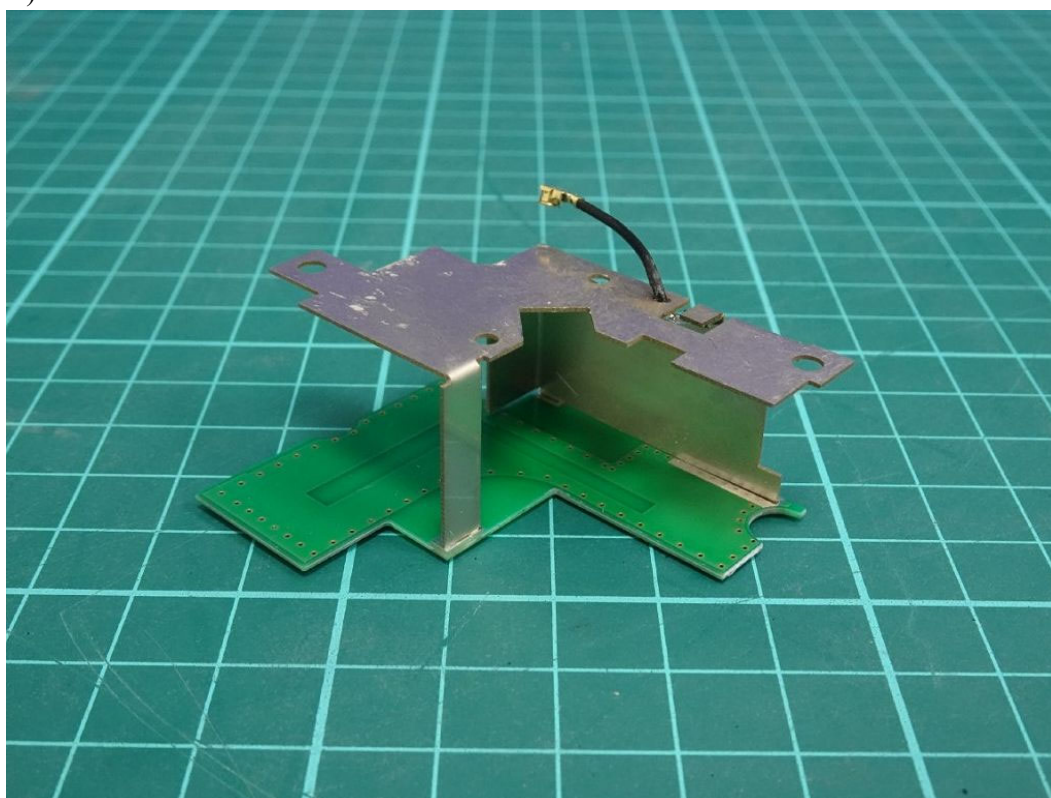
(21) EUT Photo
