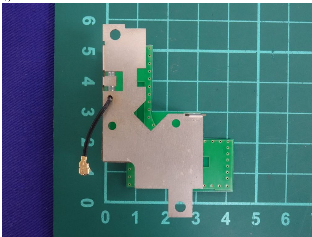
(20) EUT Photo
