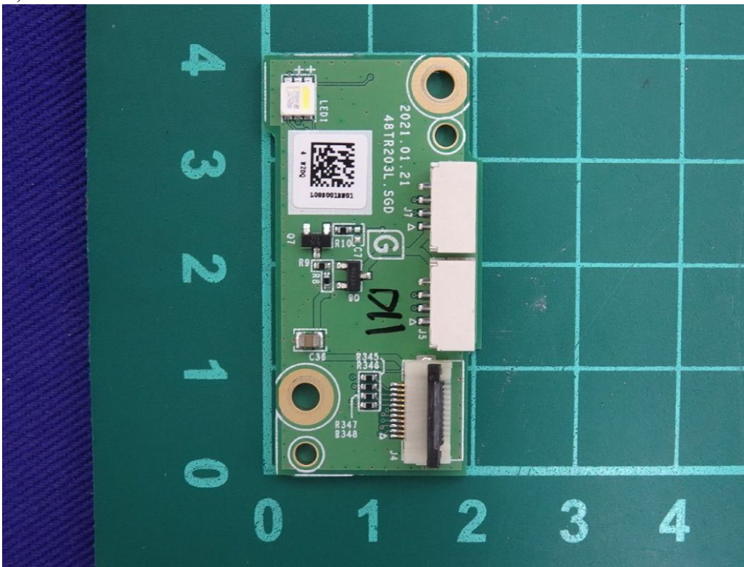
(44) EUT Photo
