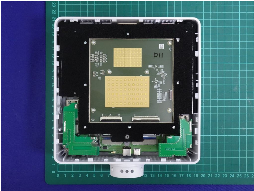
(9) EUT Photo
