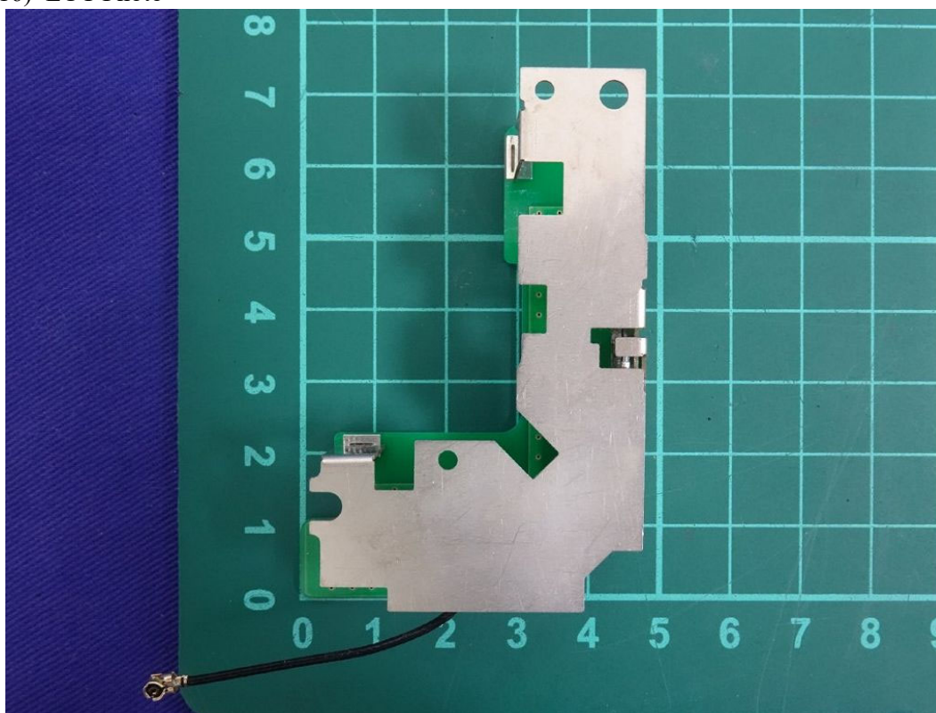
(16) EUT Photo
