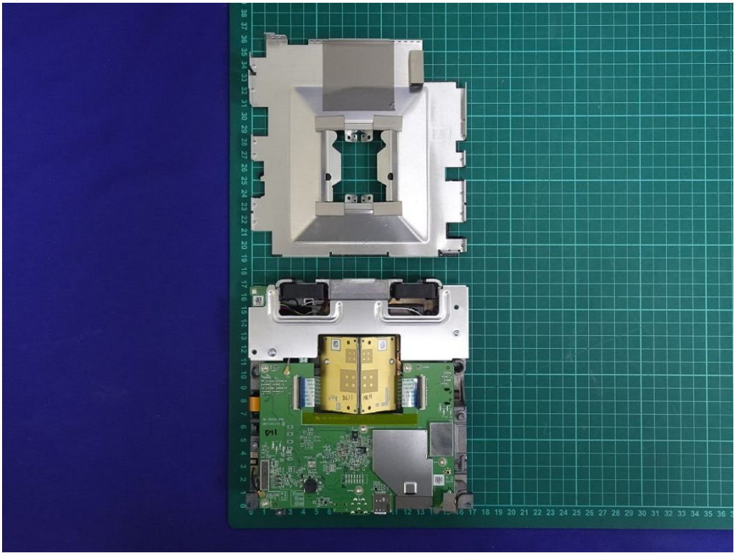
(37) EUT Photo
