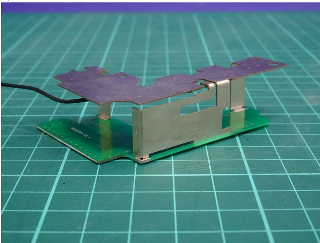
(18) EUT Photo
