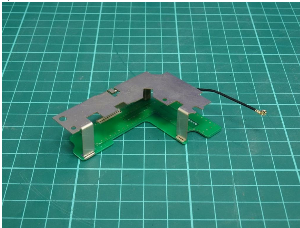
(17) EUT Photo
