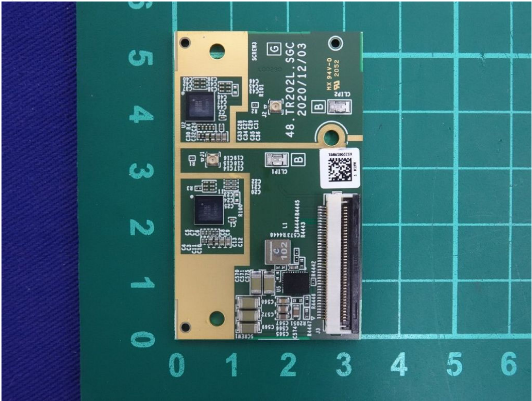
(46) EUT Photo
