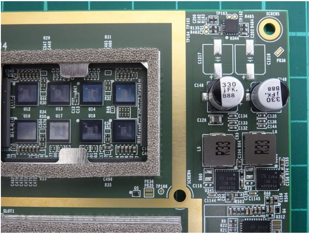
(33) EUT Photo
